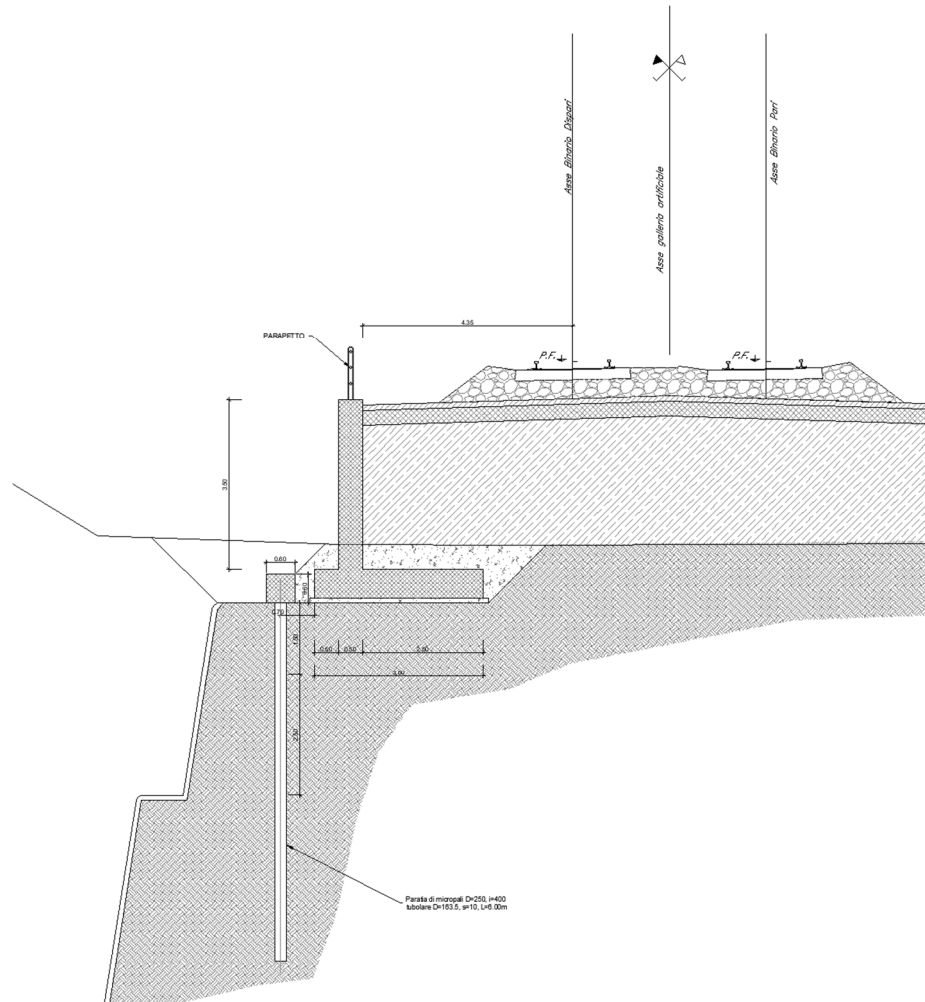
Fig. 2 – Sezione trasversale dell'opera
