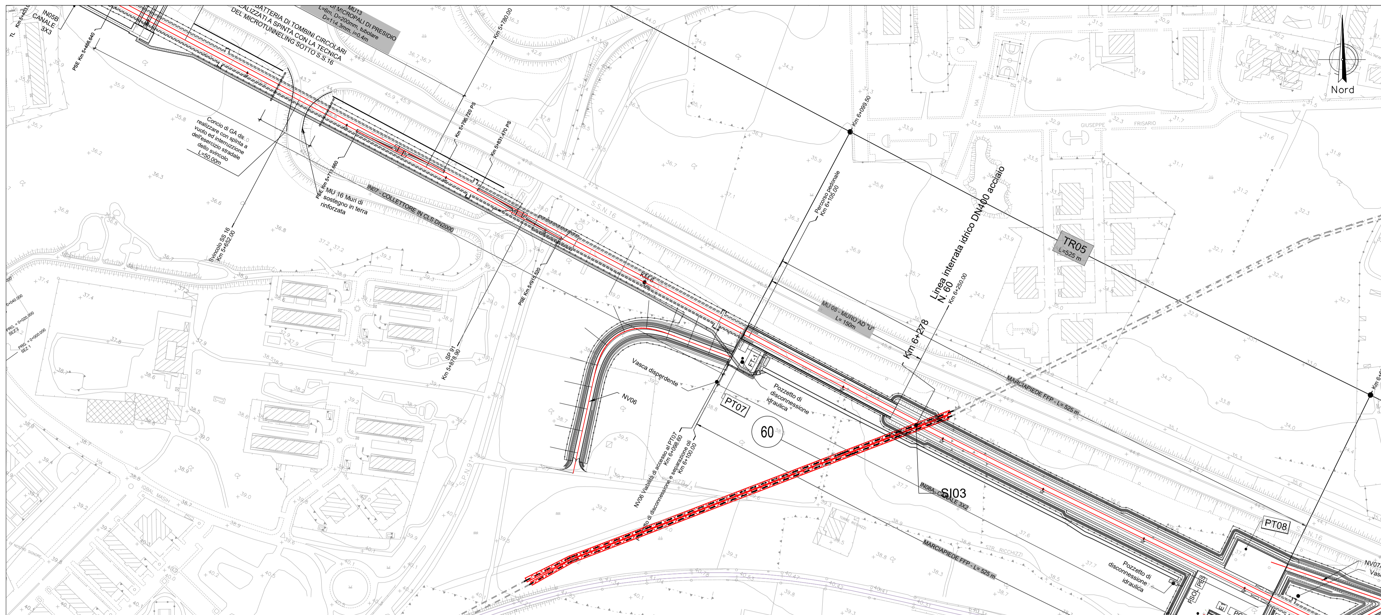
PLANIMETRIA PLANIMETRIA RISOLUZIONE INTERFERENZE SI03 Scala 1:2000
