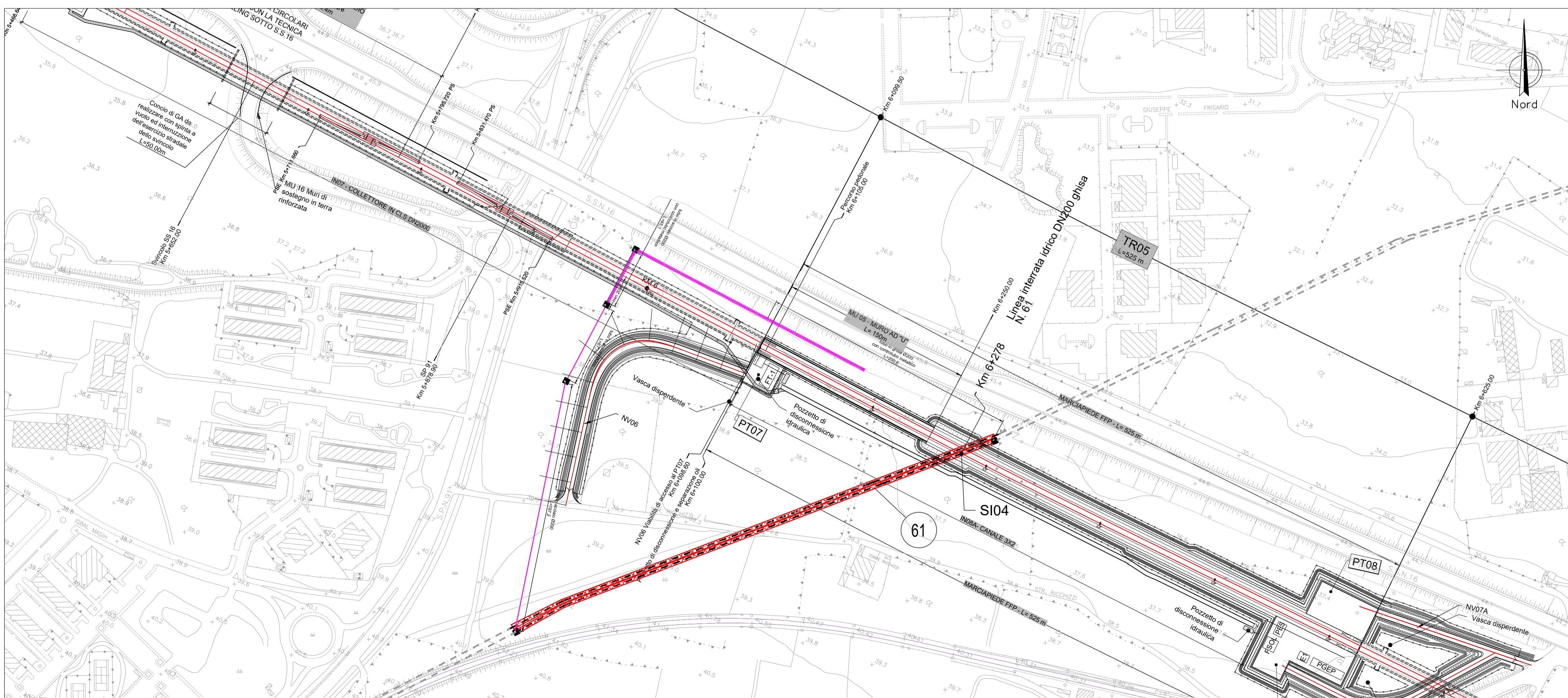
PLANIMETRIA PLANIMETRIA RISOLUZIONE INTERFERENZE SI04 Scala 1:2000
