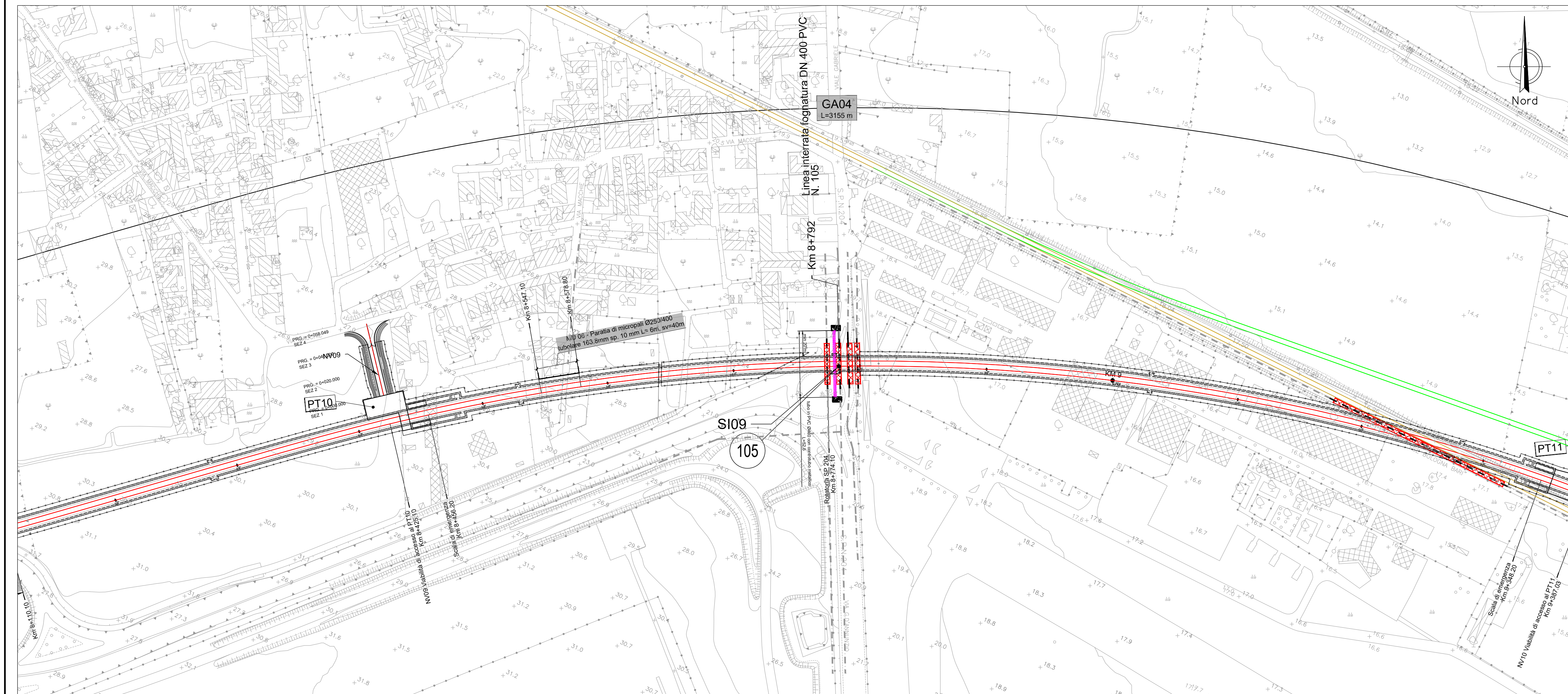
PLANIMETRIA PLANIMETRIA RISOLUZIONE INTERFERENZE SI09 Scala 1:2000
