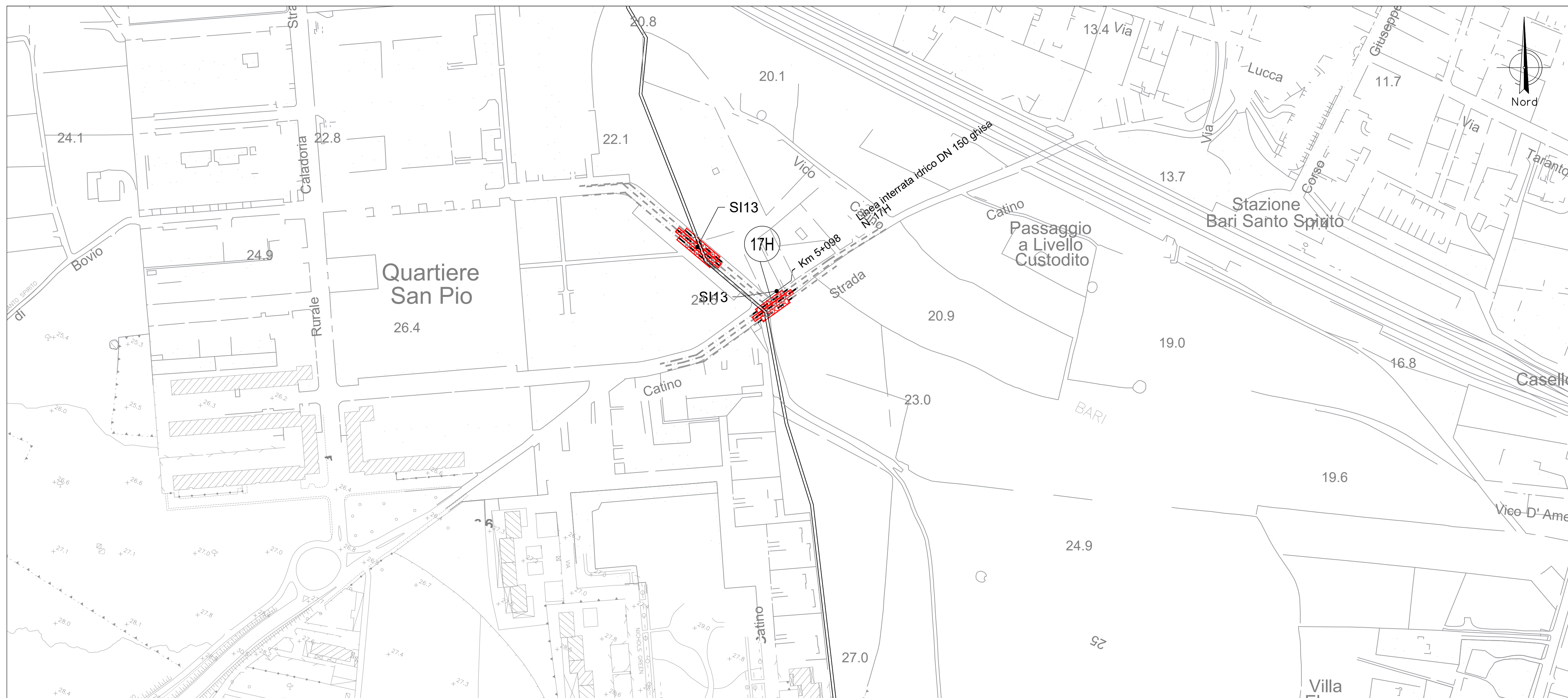
PLANIMETRIA PLANIMETRIA RISOLUZIONE INTERFERENZE SI13 Scala 1:2000
