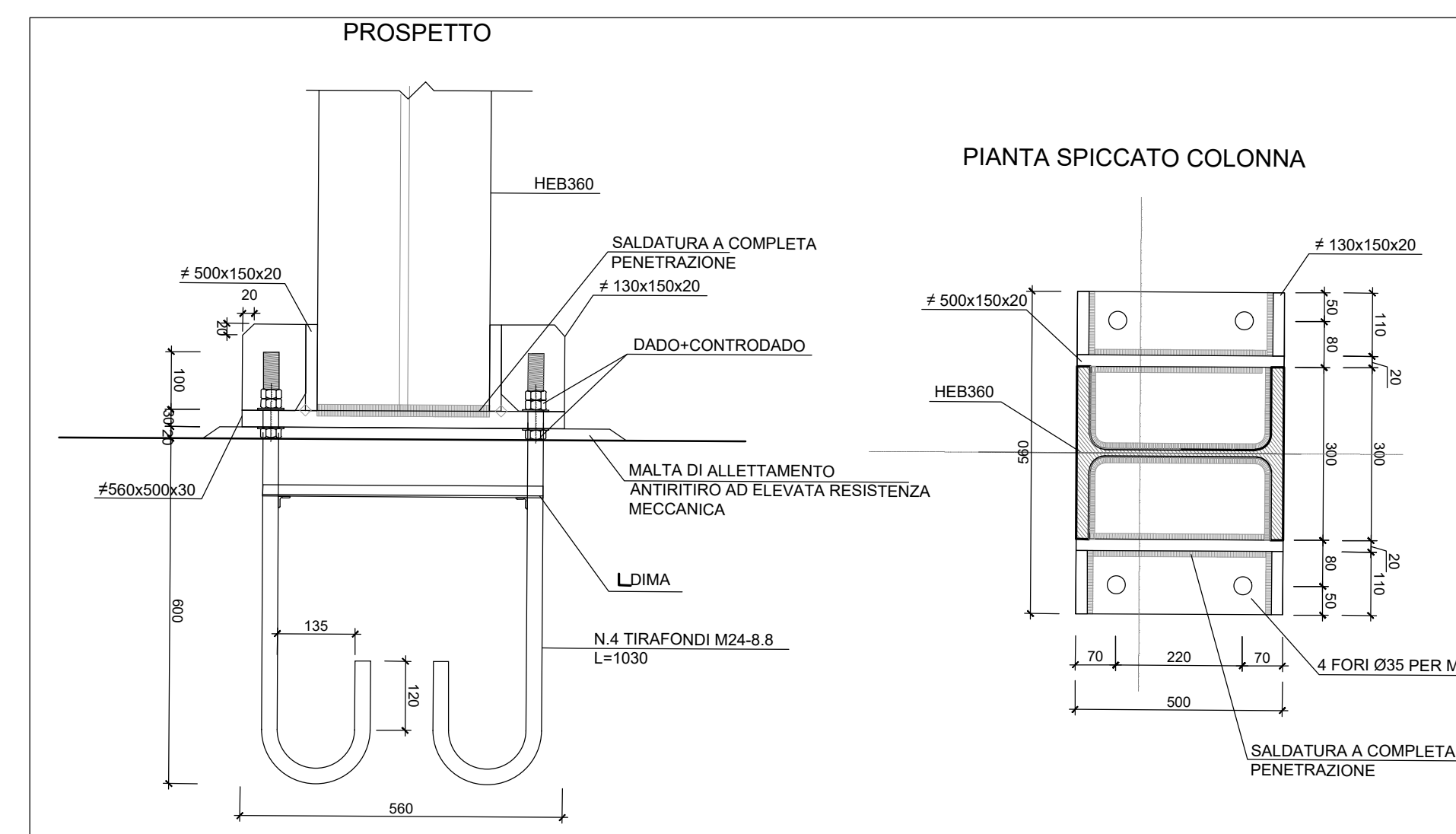
PARTICOLARE DELL' ANCORAGGIO SCALA 1:10
