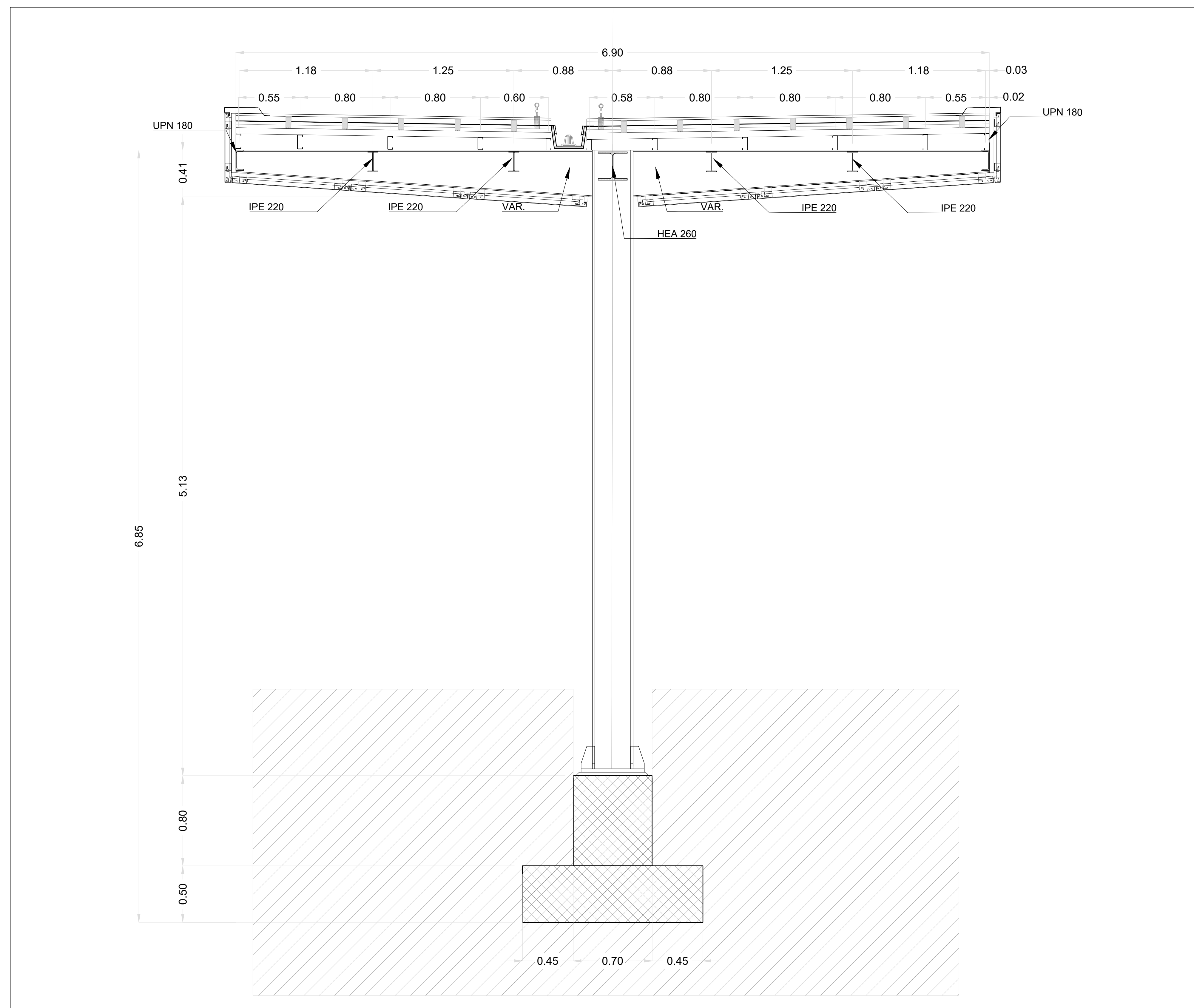
SEZIONE TRASVERSALE SCALA 1:20
