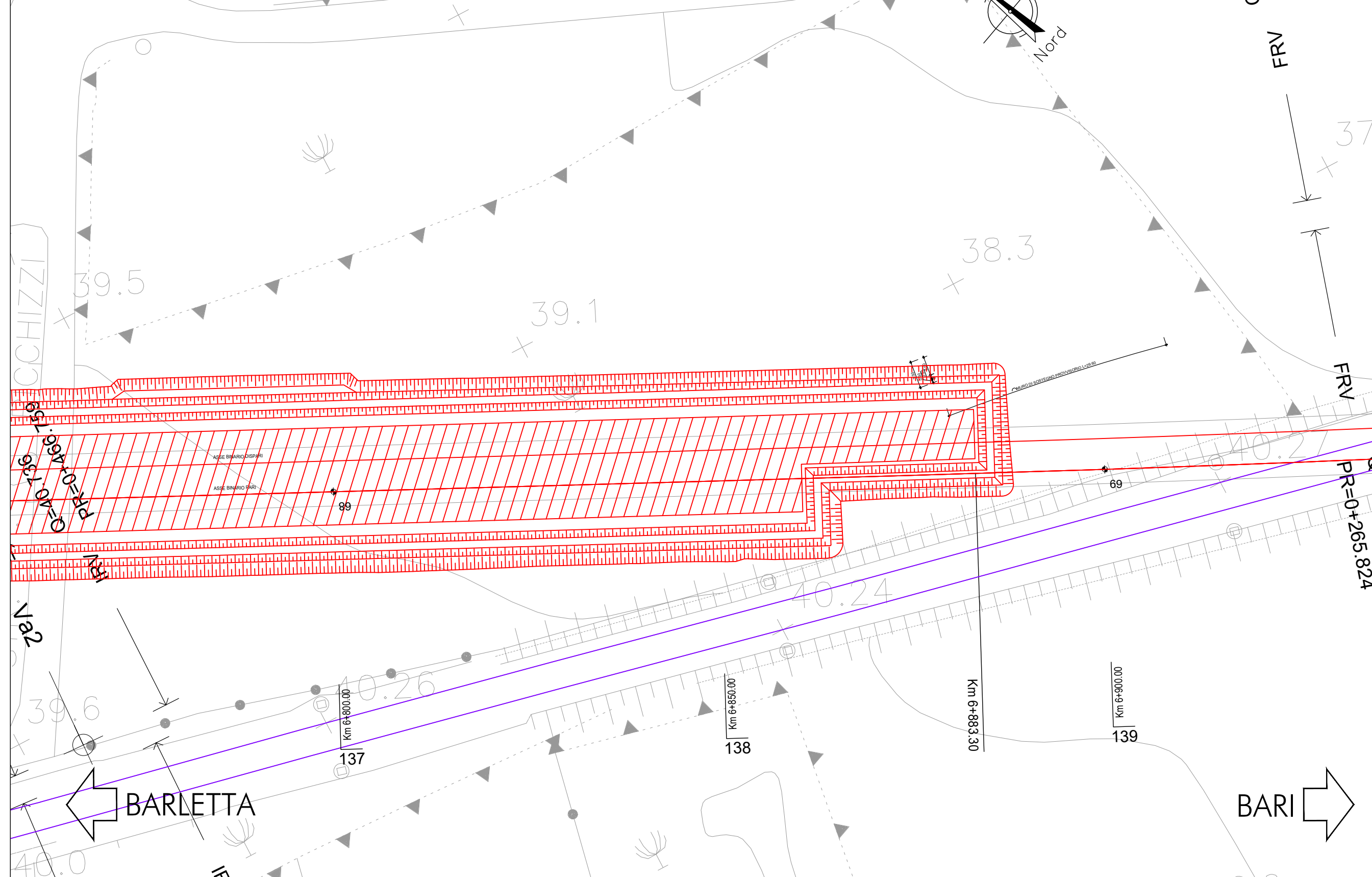
PLANIMETRIA DI PROGETTO SCALA 1:500
