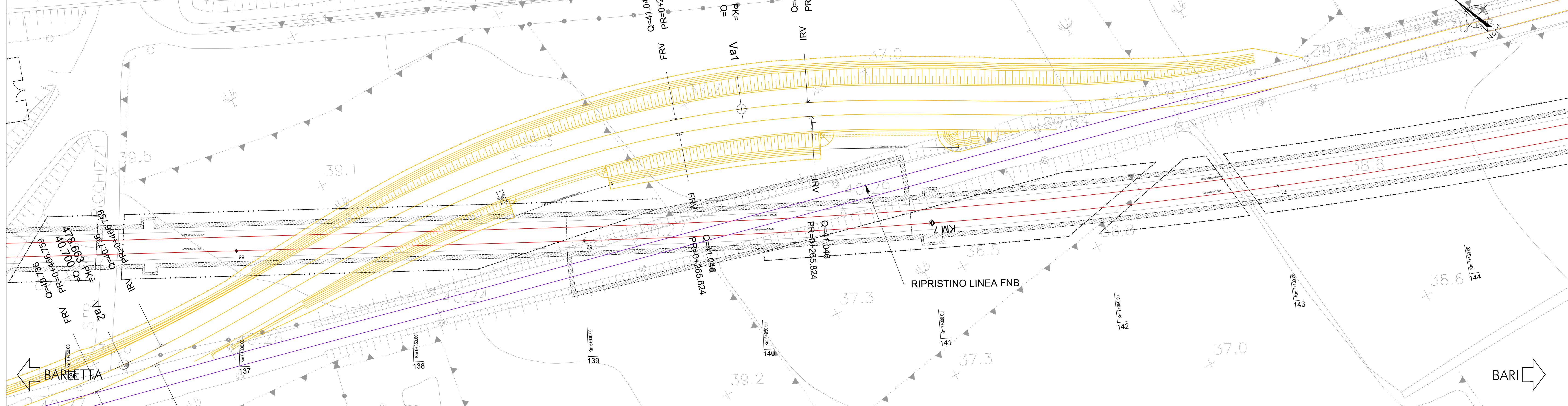
PLANIMETRIA DI PROGETTO SCALA 1:500
