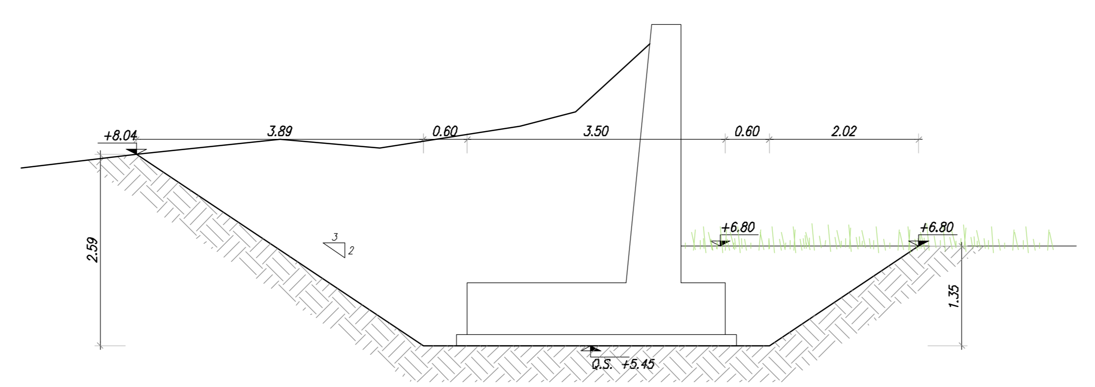
SEZIONE TRASVERSALE F-F scale 1:50
