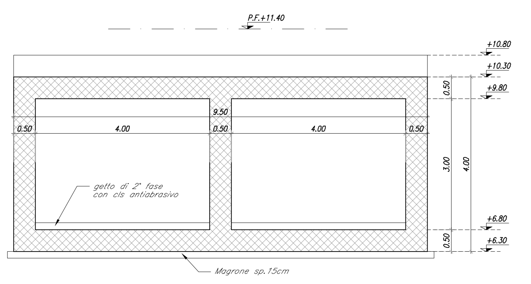
SEZIONE TRASVERSALE B-B scale 1:50
