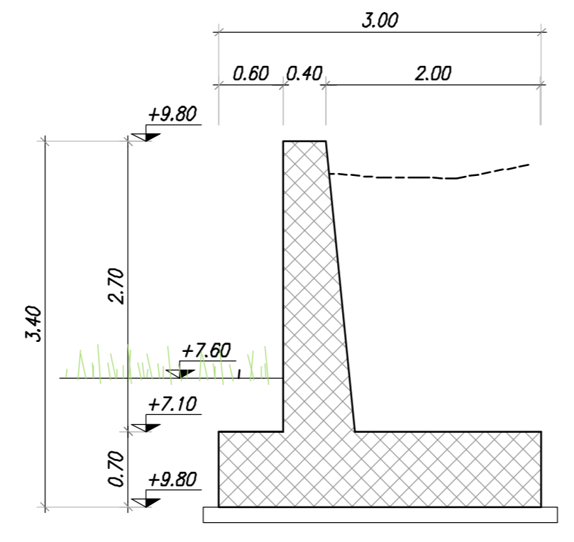
SEZIONE TRASVERSALE E-E scale 1:50
