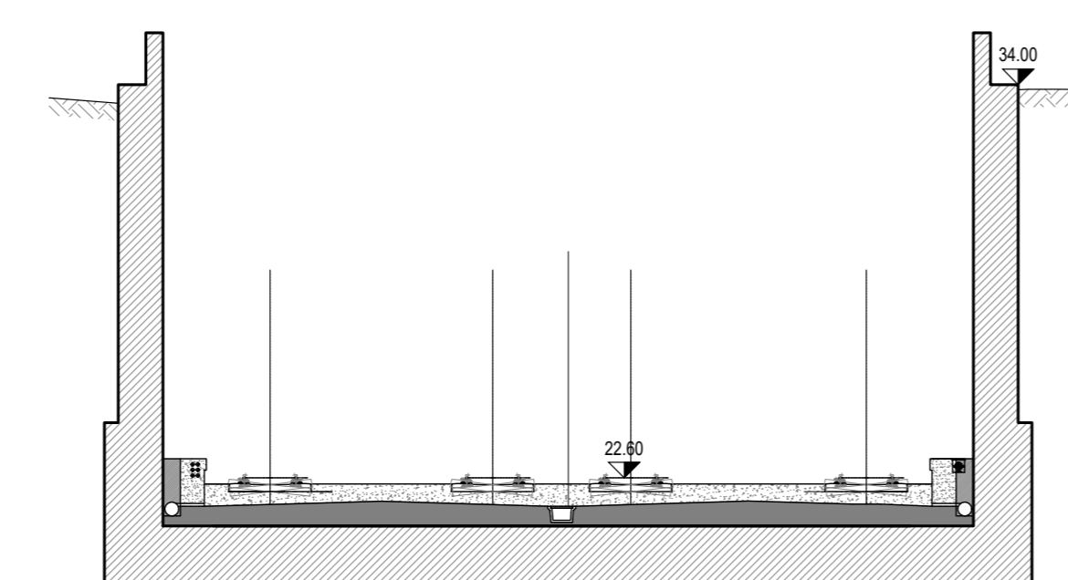
SEZIONE PK 5+250 - Scala 1:200
