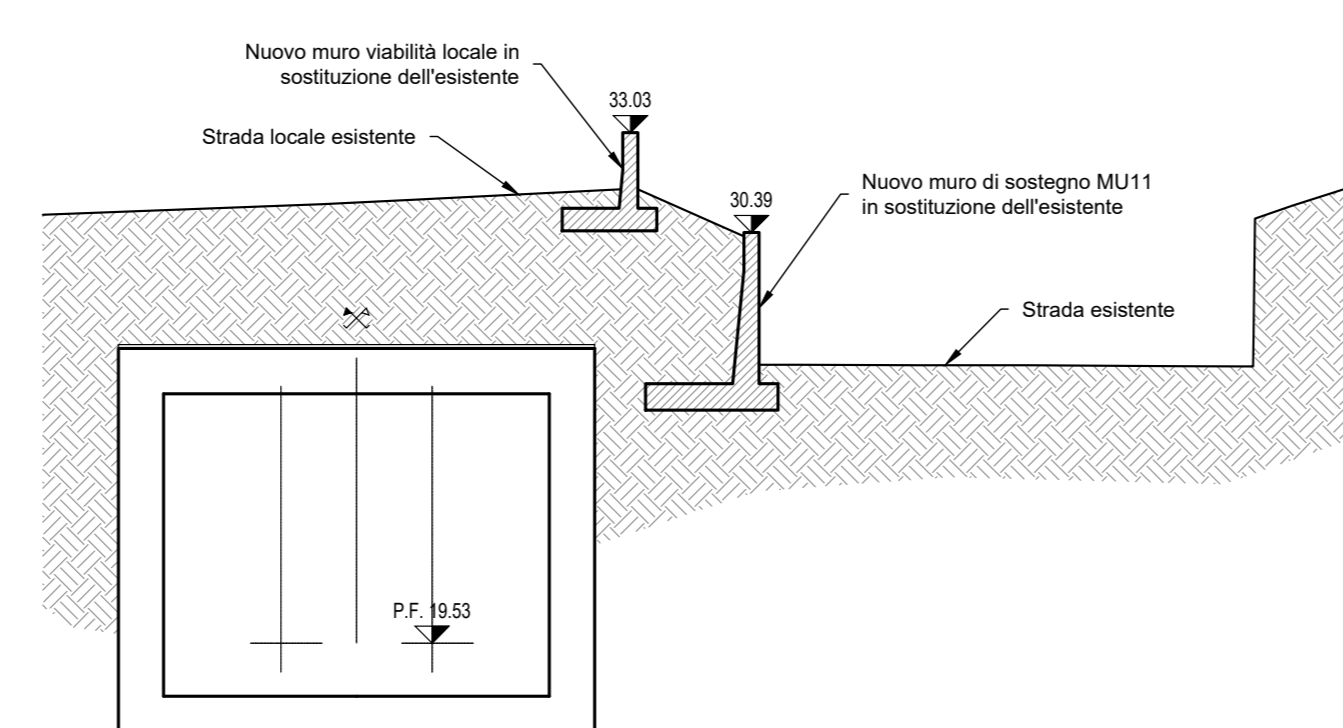
SEZIONE PK 8+075 - Scala 1:200
