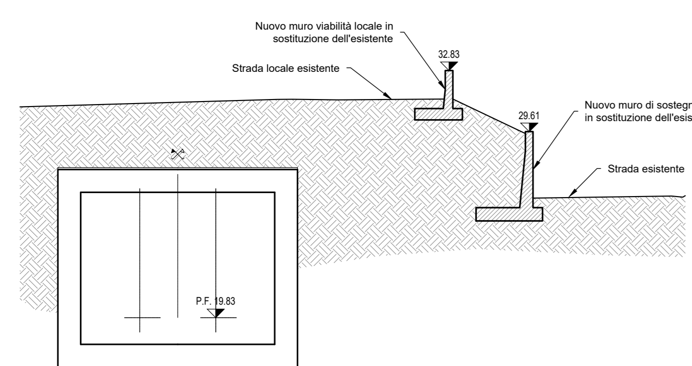
SEZIONE PK 8+050 - Scala 1:200
