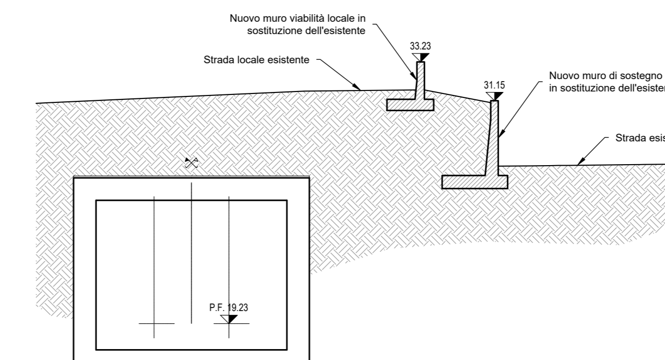
SEZIONE PK 8+100 - Scala 1:200
