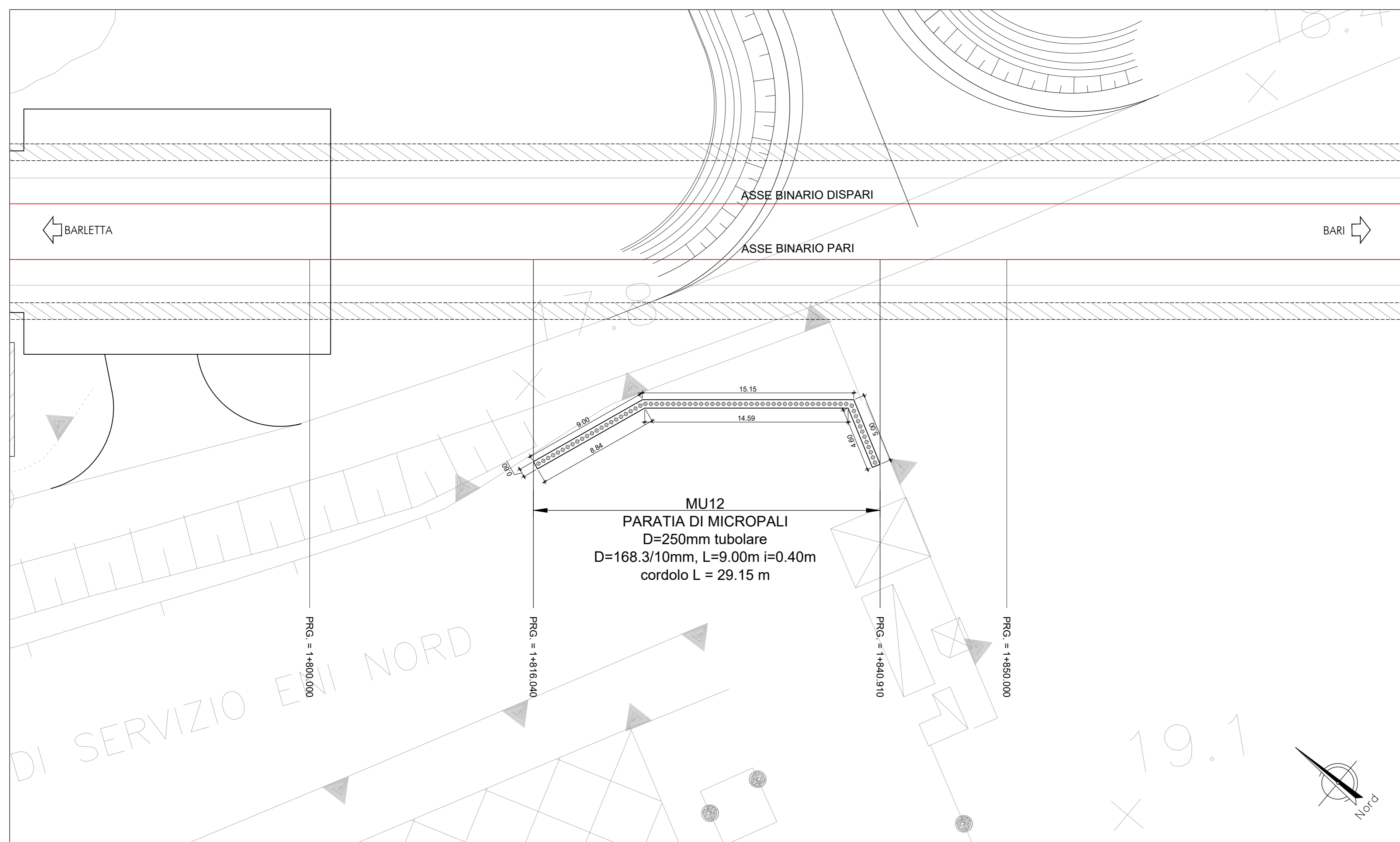
PLANIMETRIA - Scala 1:200
