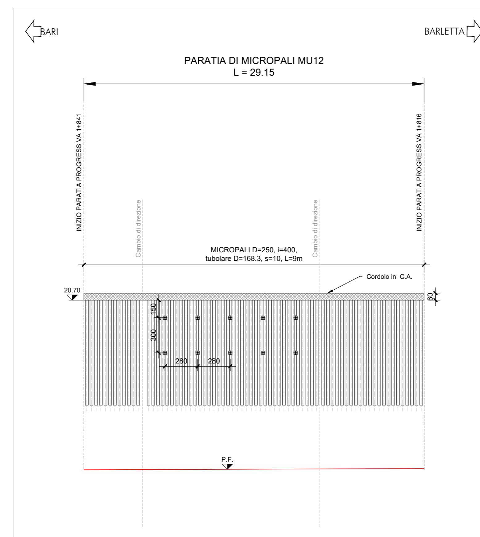
PROFILO - Scala 1:200
