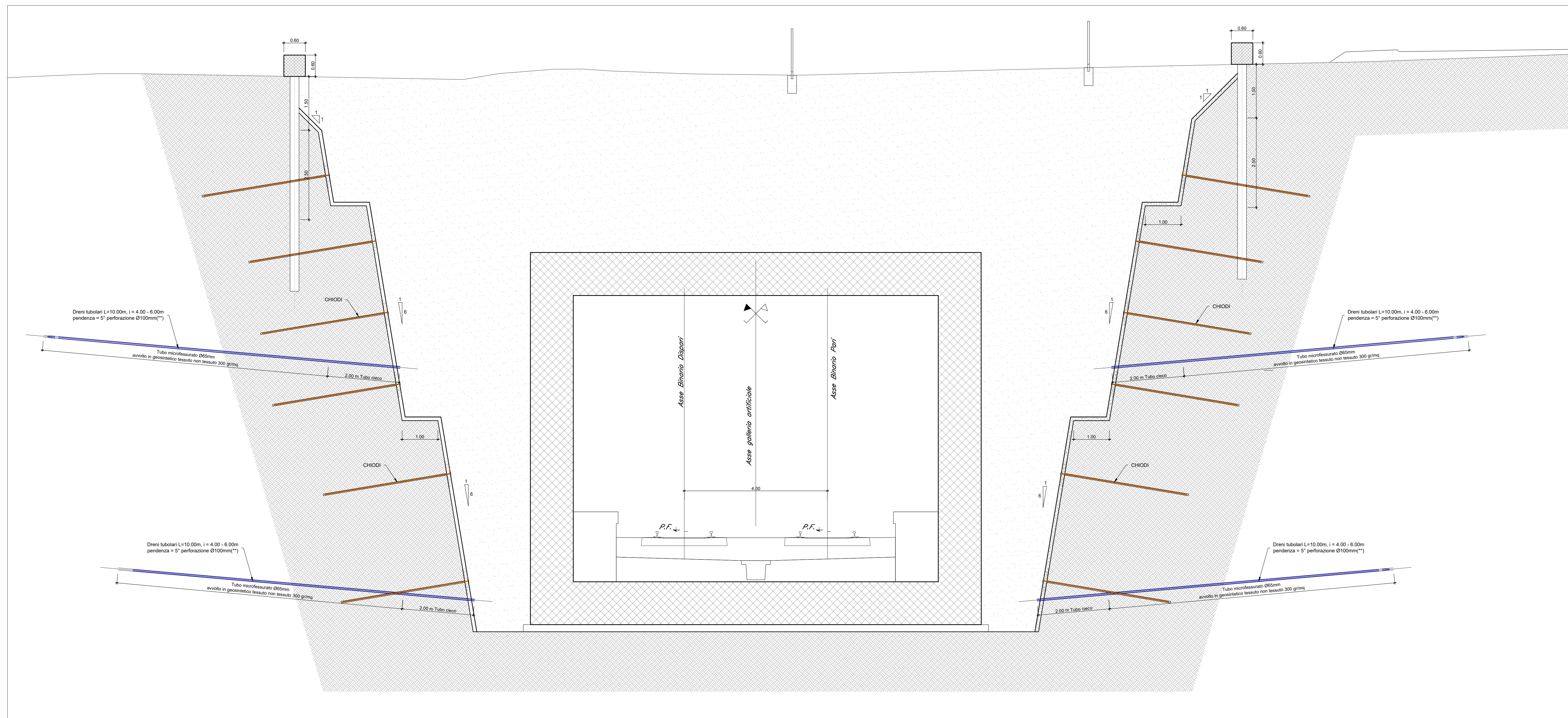
SEZIONE TIPO - Scala 1:50
