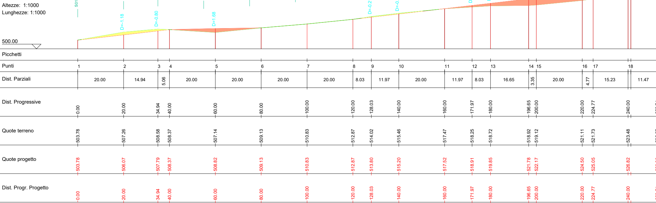
PLANIMETRIA PIAZZOLA MC03 E PROFILO C-MC03/PIAZZOLA SU CURVE DI LIVELLO_ SCALA 1:1.000
