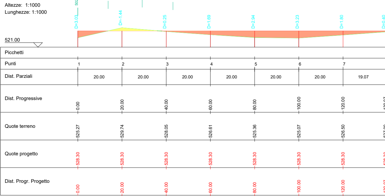
PLANIMETRIA PIAZZOLA MC03 E PROFILO C-MC03/PIAZZOLA SU CURVE DI LIVELLO_ SCALA 1:1.000
