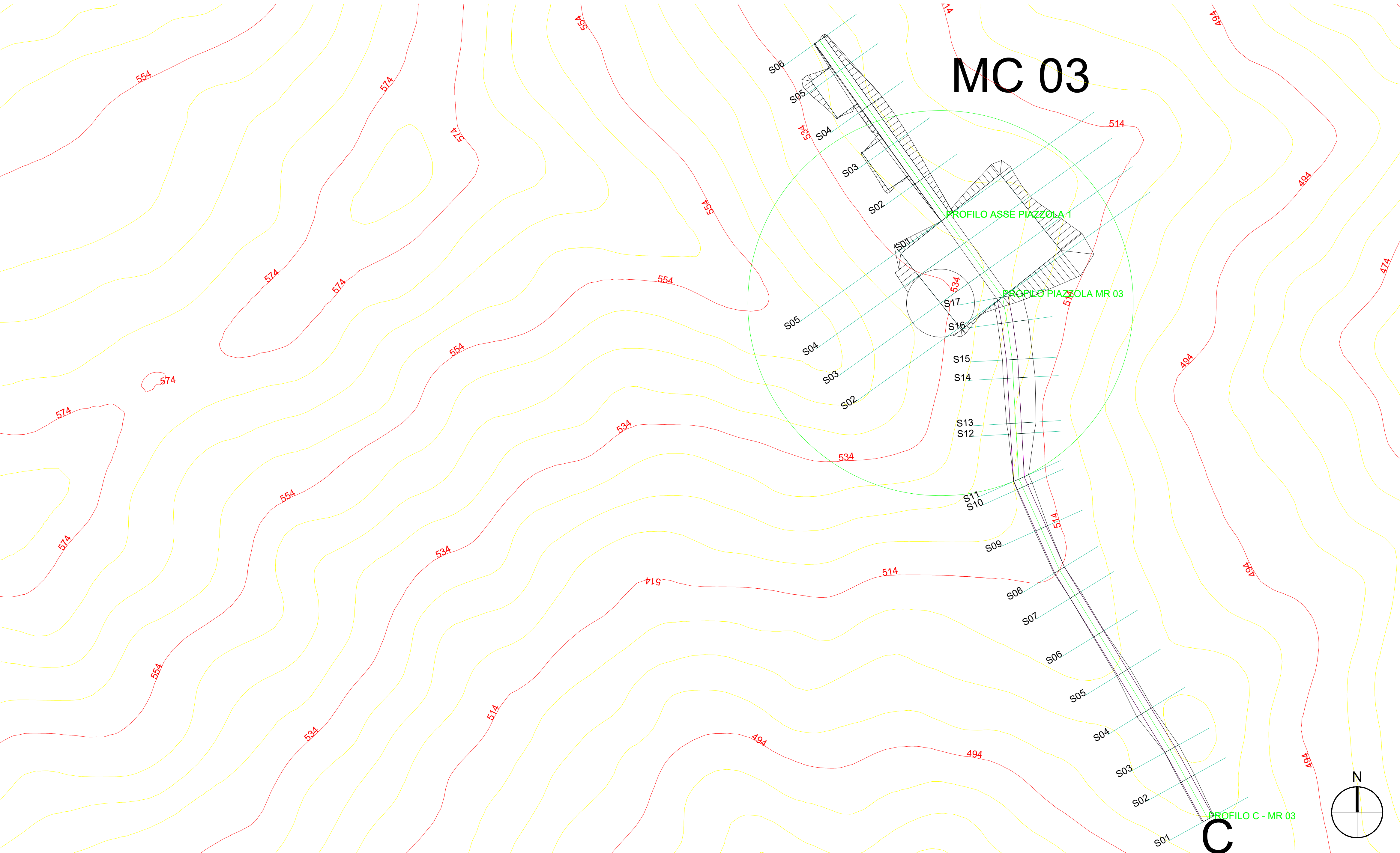
PLANIMETRIA PIAZZOLA MC03 E PROFILO C-MC03/PIAZZOLA SU CURVE DI LIVELLO_ SCALA 1:1.000
