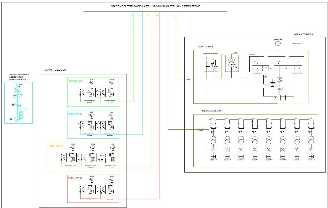
Figura 6.2.1: Schema elettrico unifilare dell’impianto utente
