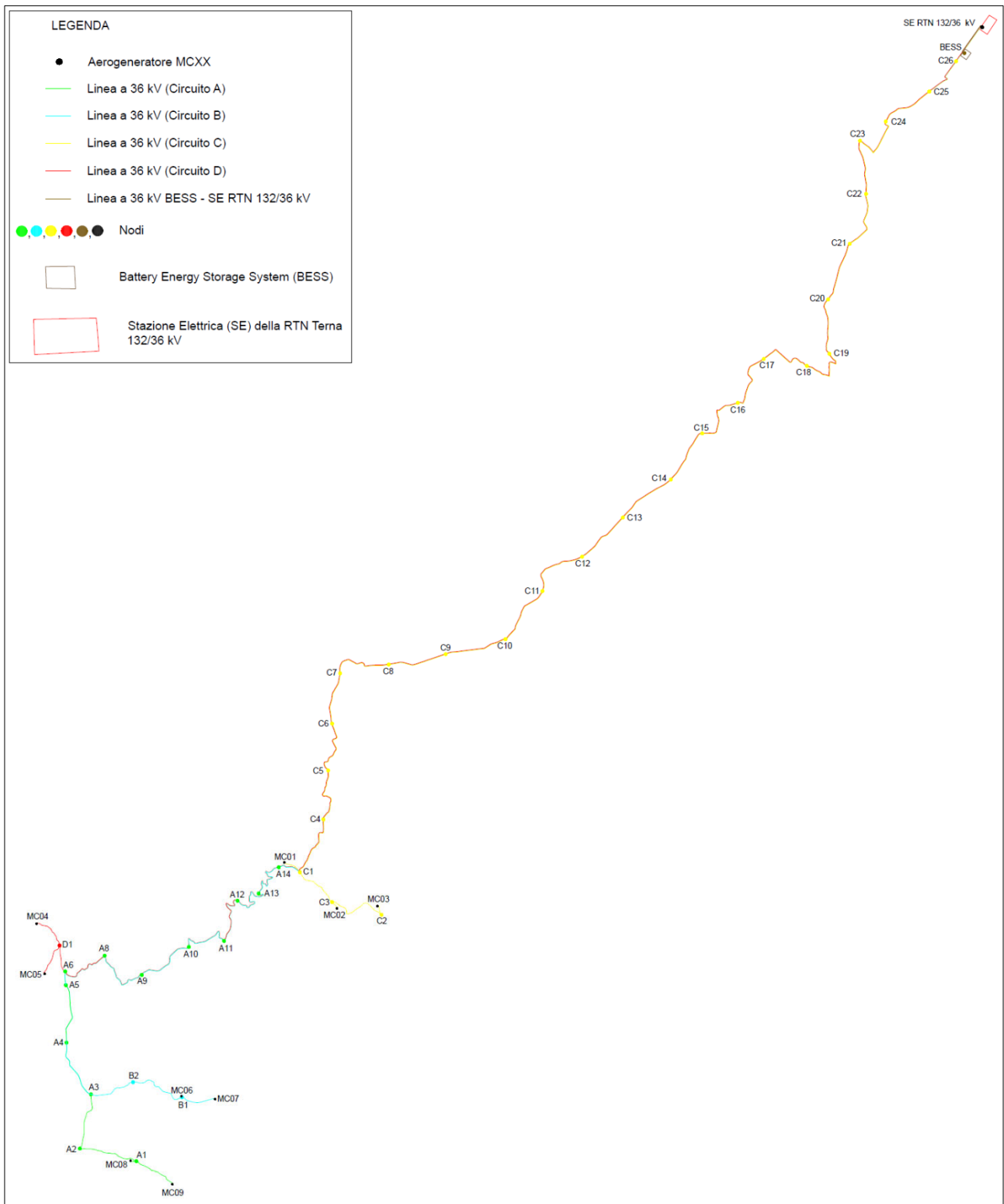
Figura 6.1.2: Planimetria di distribuzione linee a 36 kV
