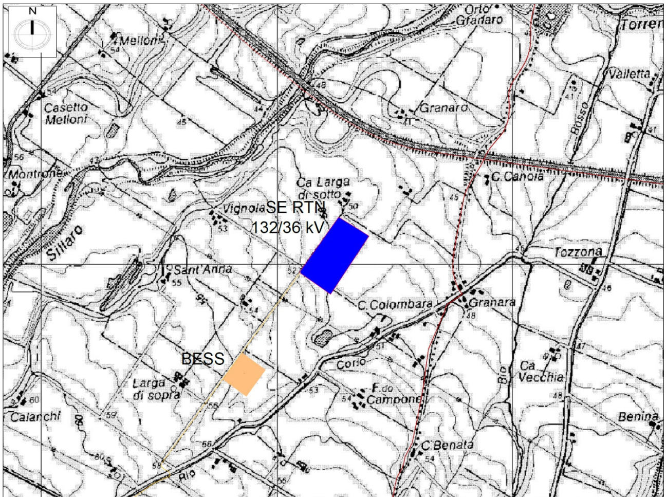
Figura 8.1.2: Ingrandimento della SE RTN 132/36 kV "Castel San Pietro" (oltre che del BESS) su CTR
