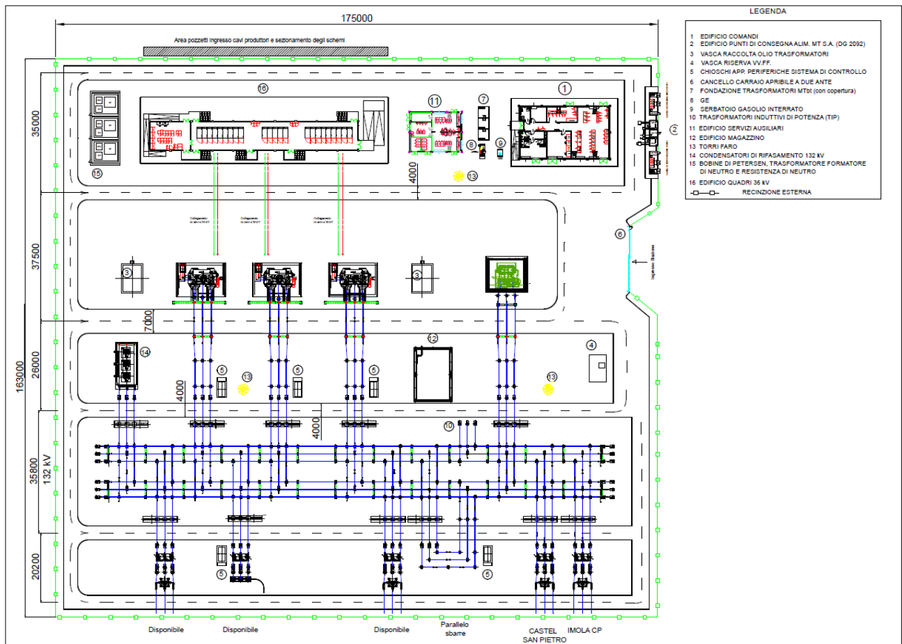
Figura 8.2.1: Planimetria elettromeccanica della stazione elettrica 132/36 kV di Castel San Pietro Terme
