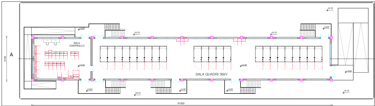
Figura 8.3.1.1: Pianta piano rialzato dell'edificio della sala quadri a 36 kV
