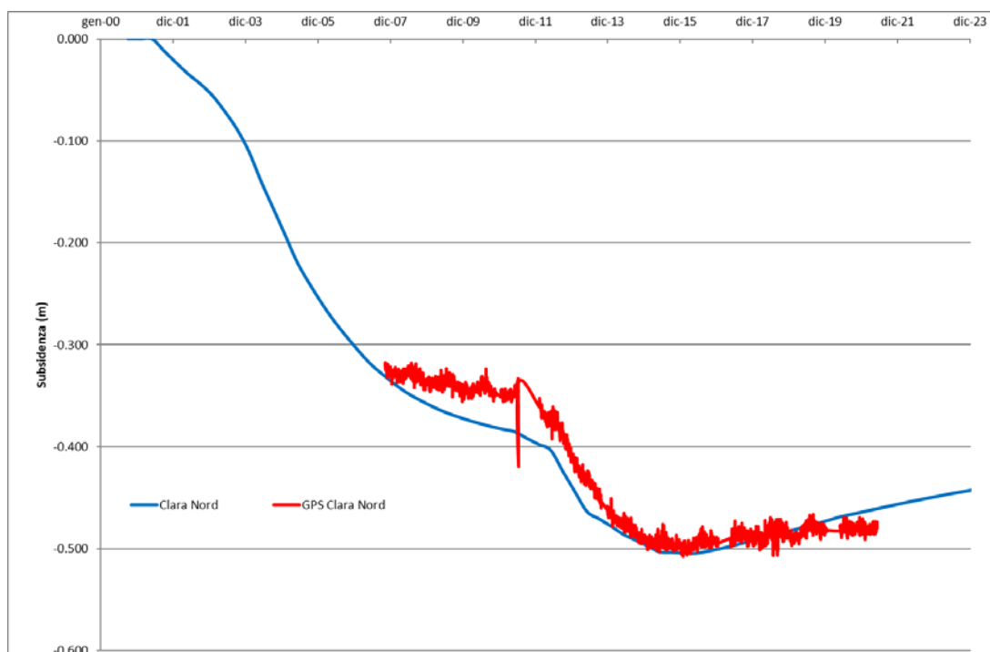
Figura 14 - Clara Nord: andamento della subsidenza misurata (CGPS in p.ma) vs. modello (scenario DN)
