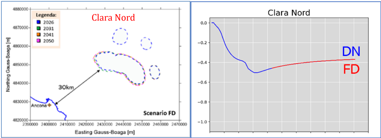
Figura 8 - Campo di Clara Nord: A sx: mappa con l'evoluzione della linea di iso-subsidenza 2 cm nel periodo 2021-2050 per lo scenario FD. La distanza minima resta pari o superiore ai 30km, e rimane pressochè invariata per l'intera durata del periodo. A dx : evoluzione della subsidenza in corrispondenza della p.ma Clara Nord nei due scenari considerati (DN e FD).
