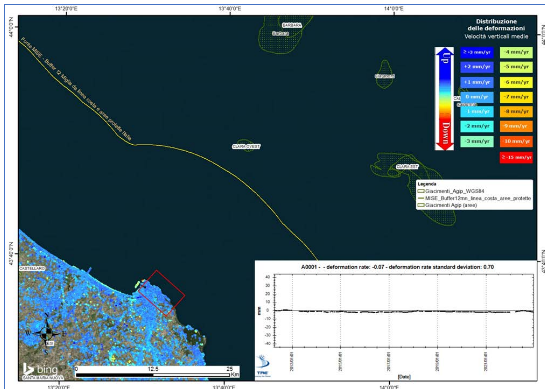
Figura 13 - Analisi dati InSAR dal 2012 al 2022 nel tratto di costa antistante il campo di Clara Nord. Serie storica media (dal 2012 al 2022) dello spostamento medio ricavata dai dati InSAR all'interno del poligono rosso.
