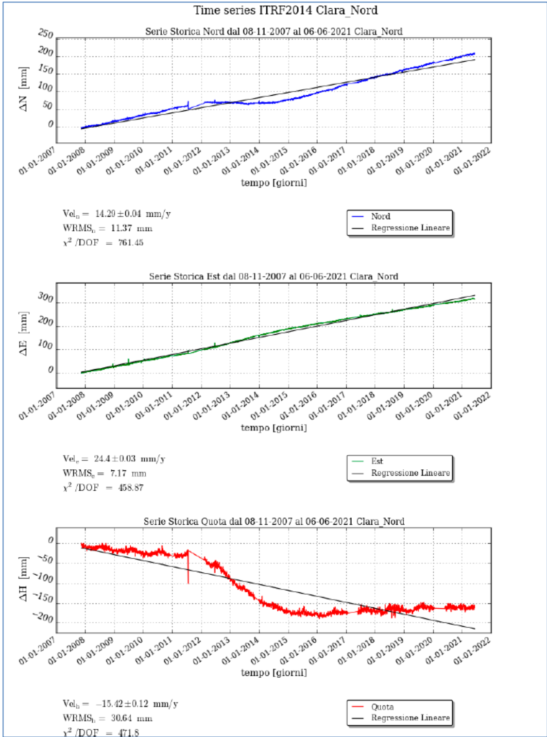
Figura 11 - Campo di Clara Nord: serie storica di misure CGPS
