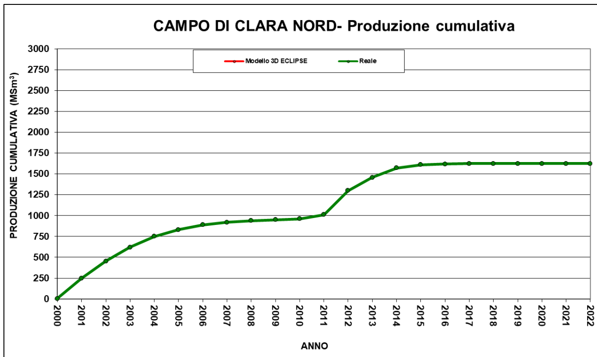
Figura 5 - Campo di Clara Nord: grafico di produzione reale e da modello Eclipse 2021
