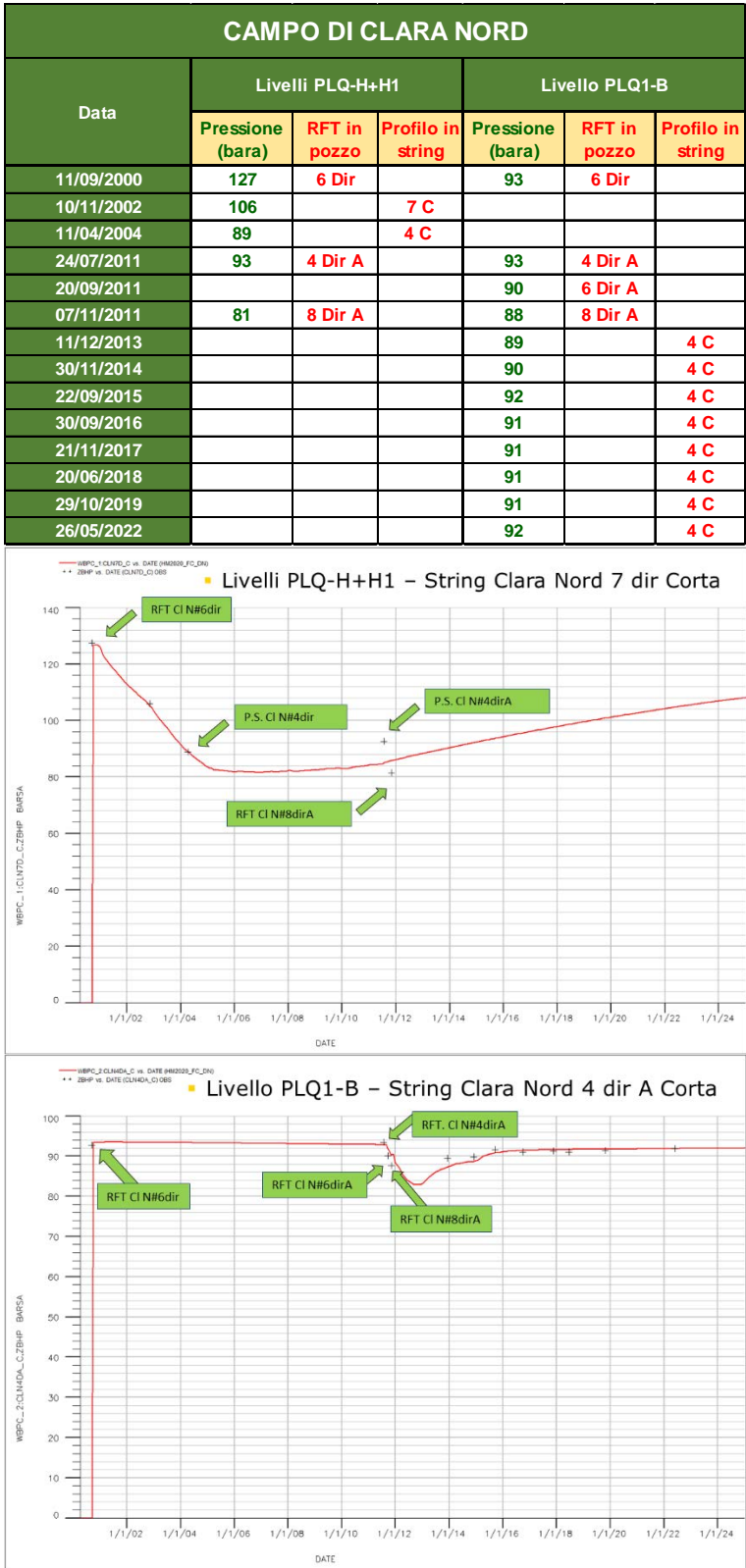
Figura 7 - Campo di Clara Nord: confronto fra i dati misurati di pressione statica e i profili di pressione calcolati da modello Eclipse 2021 - (livelli PLQ-HH1 e PLQ1-B)
