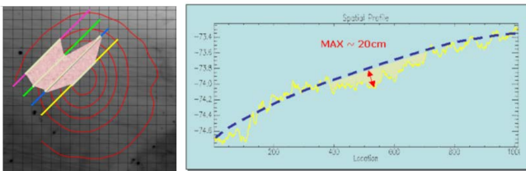
Figura 10 - Campo di Clara Nord: profilo batimetrico interpolato e differenza con la batimetria misurata
