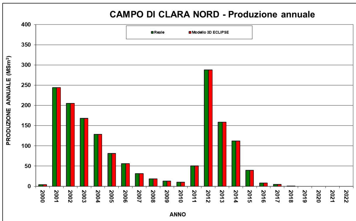
Figura 6 - Campo di Clara Nord: produzione (annuale) e da modello Eclipse 2021
