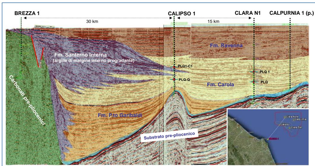
Figura 9 - Sezione sismica interpretata
