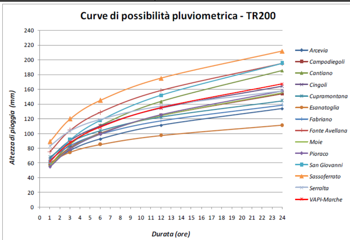
Figura 1: curve di possibilità pluviometrica (CPP), per un tempo di ritorno di 200 anni, ricavate dall'applicazione della metodologia Va.P.I. – Regione Marche ed elaborate per le stazioni pluviometriche di riferimento
