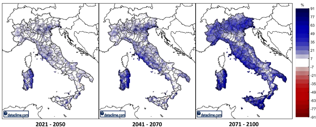
Figura 10: RCP 8.5 – Previsione del 95° percentile della precipitazione. In aggiunta all'indicatore R20, che restituisce una misura della frequenza delle precipitazioni intense (>20mm/giorno), si è considerato il 95° percentile della distribuzione delle precipitazioni giornaliere (R95p) come stima di "magnitudo" degli eventi, per i tre periodi previsionali 2021-2050, 2041-2070, 2071-2100. Le mappe indicano le anomalie in termini di valori medi rispetto al periodo di riferimento 1981-2010.
