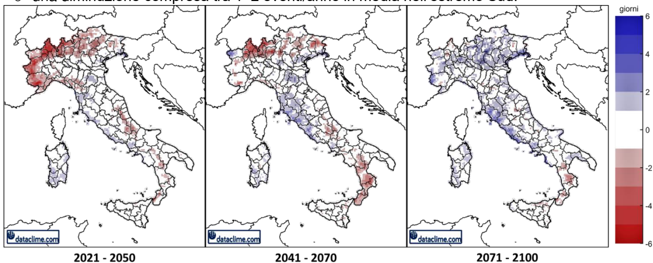
Figura 7: RCP 4.5 - Previsione dei Giorni di Precipitazioni Intense R20 (Media Annuale del numero di giorni con precipitazione giornaliera superiore ai 20 mm [unità di misura giorni/anno]) per i tre periodi previsionali 2021-2050, 2041-2070, 2071-2100. Le mappe indicano le anomalie in termini di valori medi rispetto al periodo di riferimento 1981-2010.
