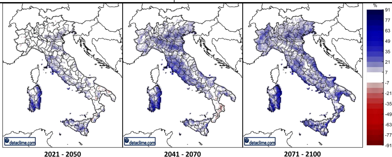
Figura 9: RCP 4.5 – Previsione del 95° percentile della precipitazione. In aggiunta all'indicatore R20, che restituisce una misura della frequenza delle precipitazioni intense (>20mm/giorno), si è considerato il 95° percentile della distribuzione delle precipitazioni giornaliere (R95p) come stima di "magnitudo" degli eventi, per i tre periodi previsionali 2021-2050, 2041-2070, 2071-2100. Le mappe indicano le anomalie in termini di valori medi rispetto al periodo di riferimento 1981-2010.
