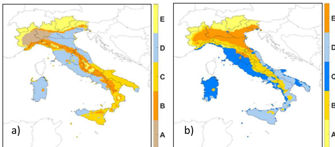
Figura 11: Mappa dei cluster individuati - a) Scenario RCP4.5; b) Scenario RCP8.5
