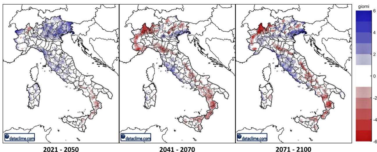
Figura 8: RCP 8.5 – Previsione dei Giorni di Precipitazioni Intense R20 (Media Annuale del numero di giorni con precipitazione giornaliera superiore ai 20 mm [unità di misura giorni/anno]) per i tre periodi previsionali 2021-2050, 2041-2070, 2071-2100. Le mappe indicano le anomalie in termini di valori medi rispetto al periodo di riferimento 1981-2010.
