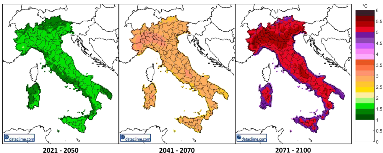
Figura 6: RCP 8.5 – Previsione della Media annuale della temperatura media giornaliera [°C], per i tre periodi previsionali 2021-2050, 2041-2070, 2071-2100. Le mappe indicano le anomalie in termini di valori medi rispetto al periodo di riferimento 1981-2010.
