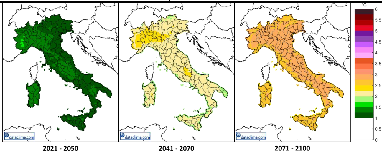
Figura 5: RCP 4.5 – Previsione della Media annuale della temperatura media giornaliera [°C], per i tre periodi previsionali 2021-2050, 2041-2070, 2071-2100. Le mappe indicano le anomalie in termini di valori medi rispetto al periodo di riferimento 1981-2010.
