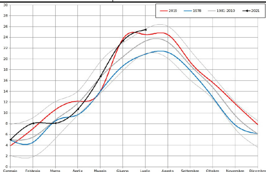
Figura 2: andamento temperatura media mensile regionale (°C); in nero l'anno attuale, in rosso l'anno più caldo dal 1961, in blu l'anno più freddo dal 1961, in grigio la media 1981-2010 ed i limiti rappresentati dalla media \pm due volte la deviazione standard.
