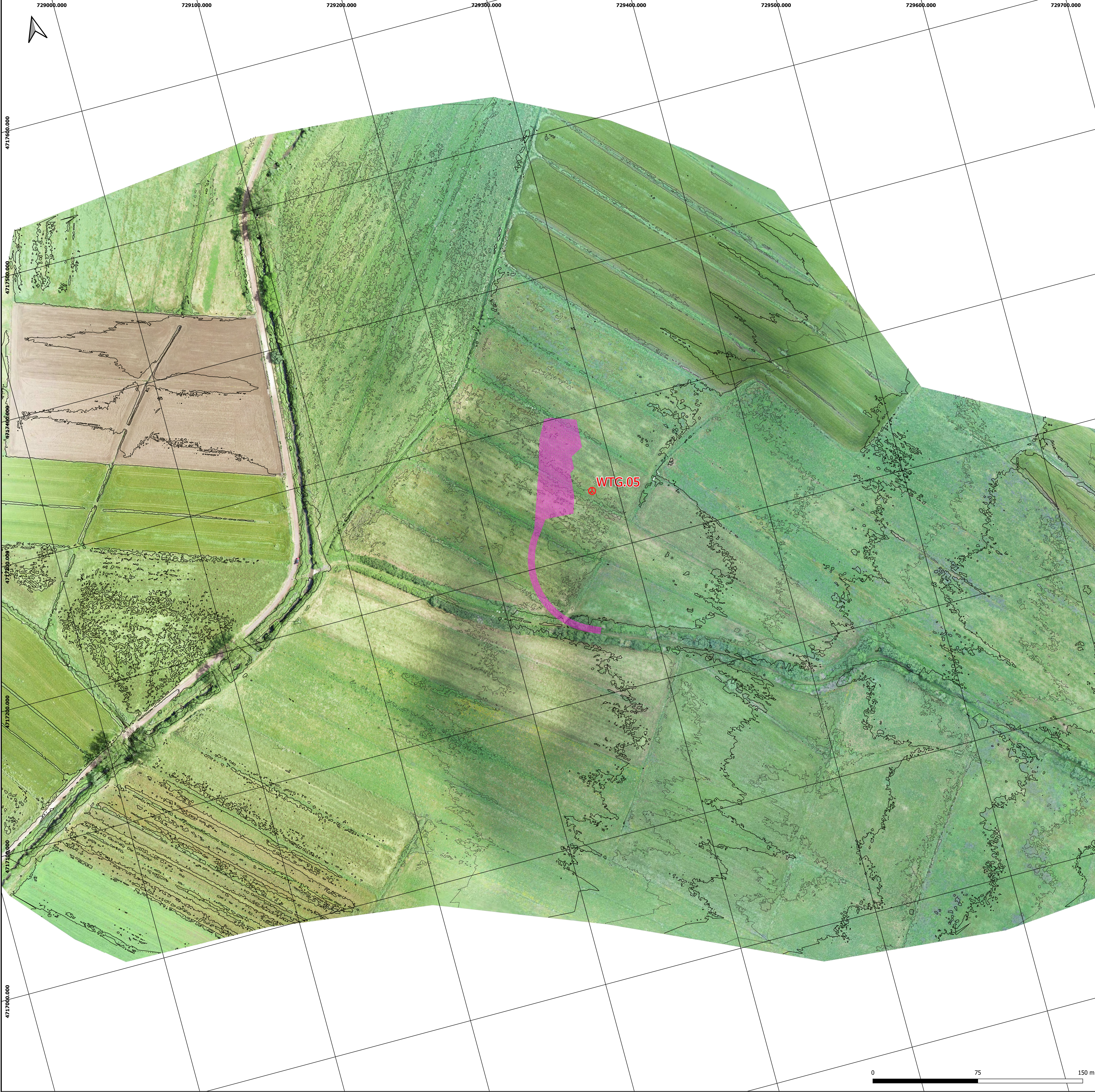
ORTOFOTO DA RILIEVO DRONE CON CURVE DI LIVELLO risoluzione foto 0.5 m/pixel - risoluzione DTM 0.5 m/pixel AREA WTG.05
