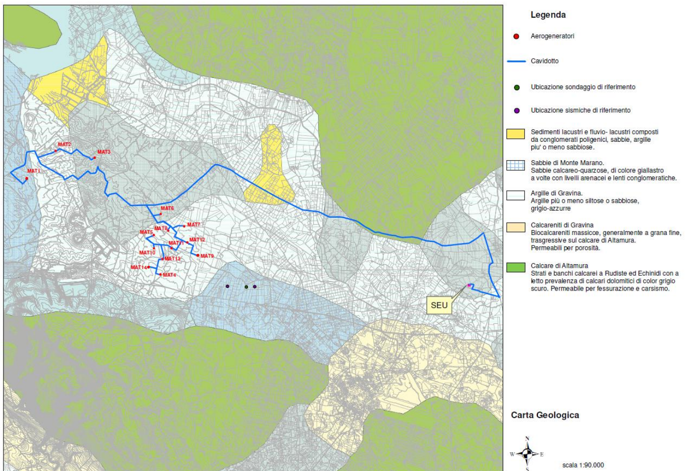
Figura 4.3-1: Stralcio Carta Geologica – Foglio 189 e 201
