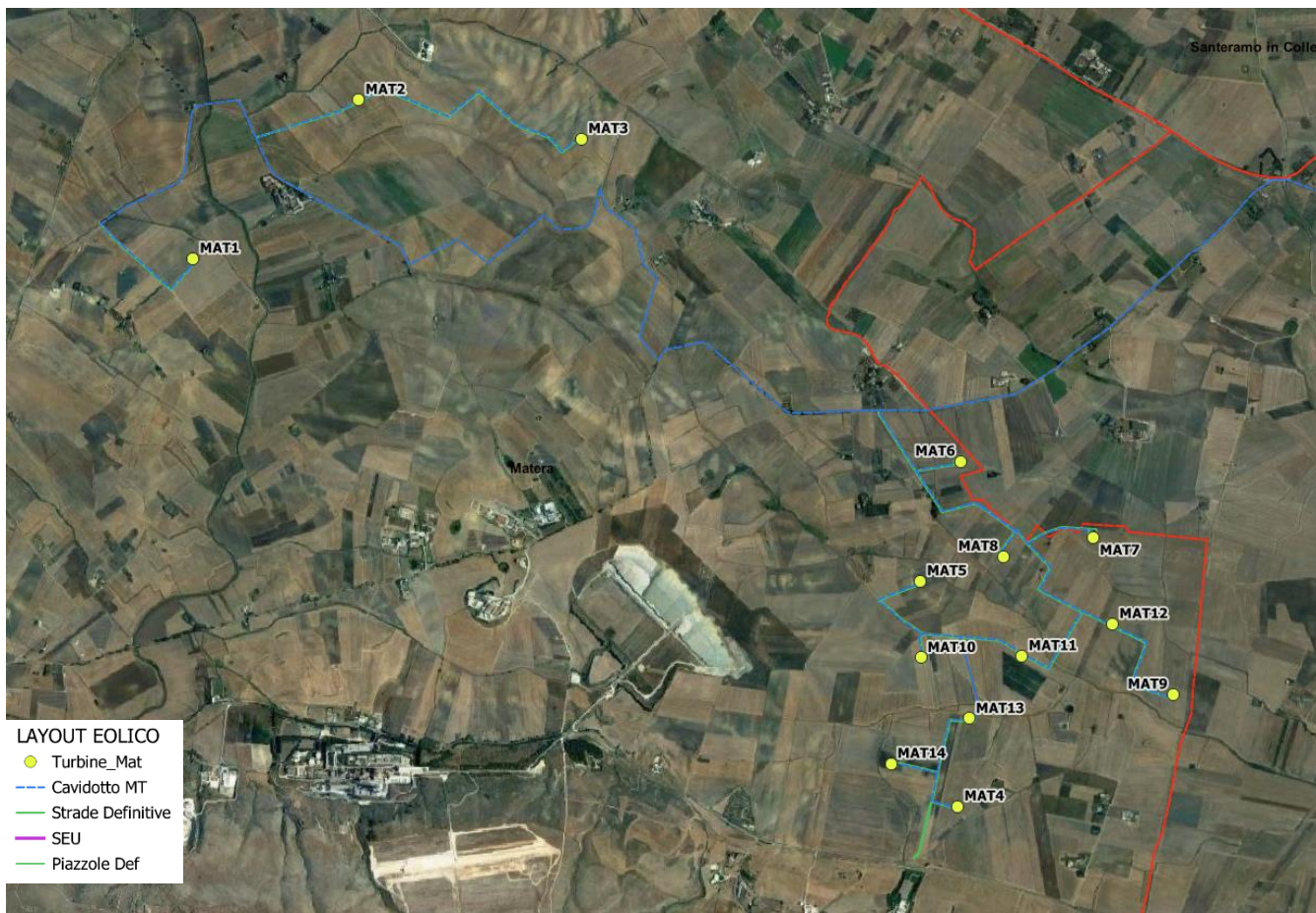
Figura 2.1-4: Area di sito: dettaglio layout di progetto su ortofoto
