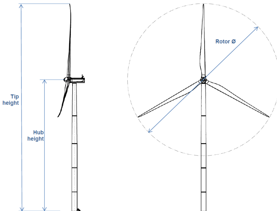
Figura 2.3-1: Struttura aerogeneratore
