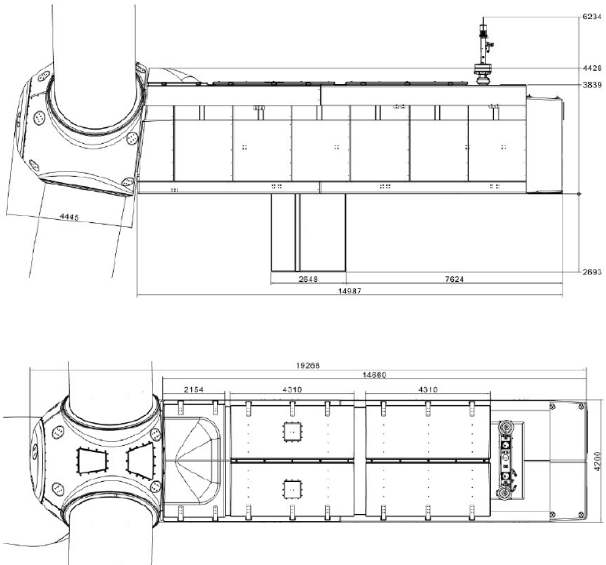
Figura c-2: Tipico navicella
