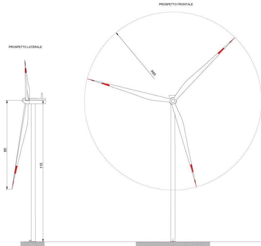
Figura c-1: Struttura aerogeneratore
