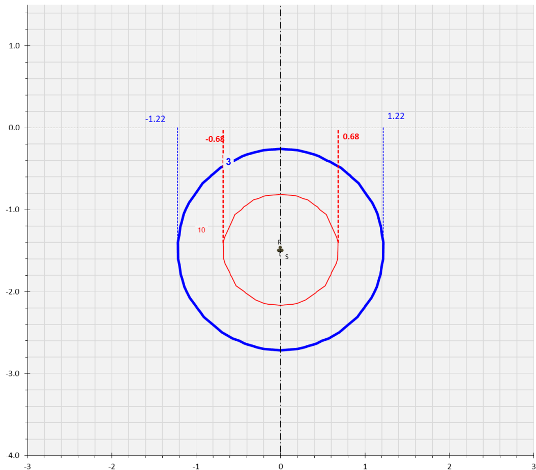
Figura 5: Curve di equilivello per il campo di induzione magnetica generato dalla linea AT (Sezione 1 – una terna AT)
