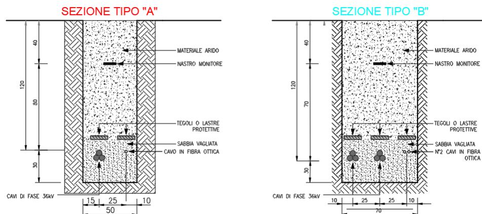
Figura 1: Sezioni tipiche di posa della linea in cavo su strade sterrate e terreno agricolo
