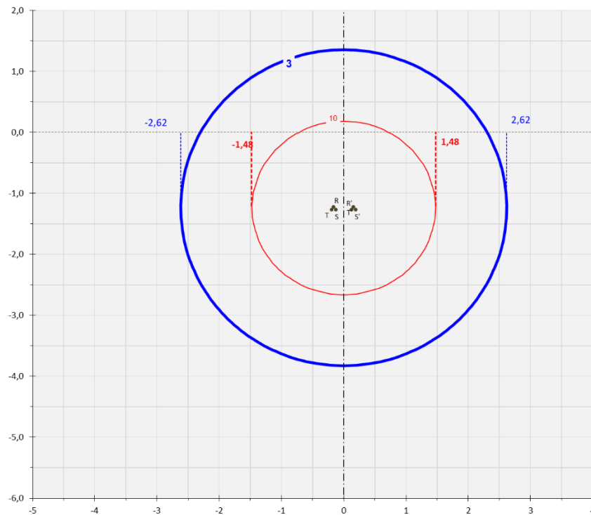
Figura 6: Curve di equilivello per il campo di induzione magnetica generato dalla linea (Sezione 2 – due terne a 36 kV)
