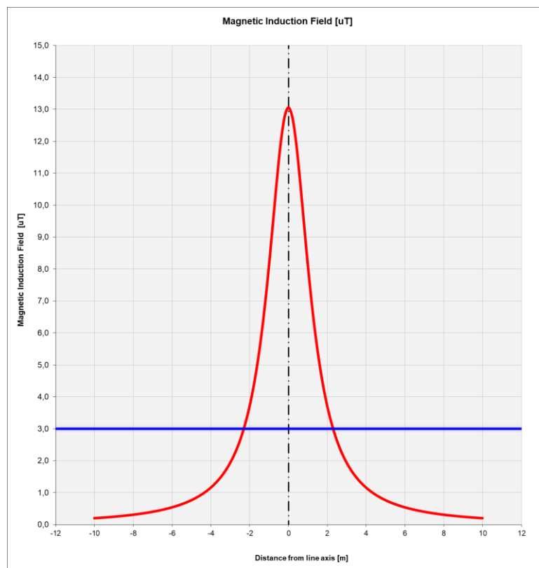
Figura 4: Andamento dell'induzione magnetica prodotta dalla linea in cavo per la sezione 2 (due terne a 36 kV)
