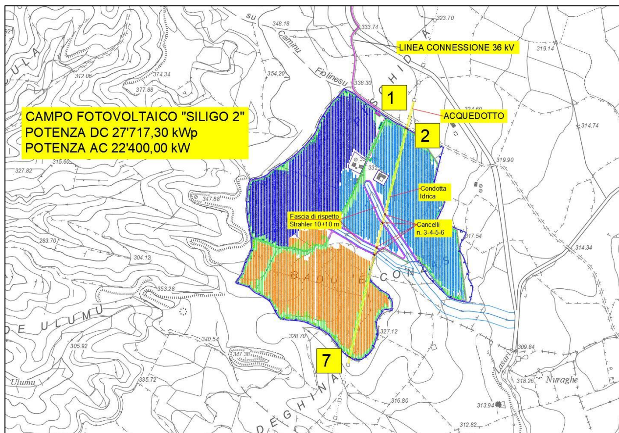
Fig. 1 Area d'impianto
