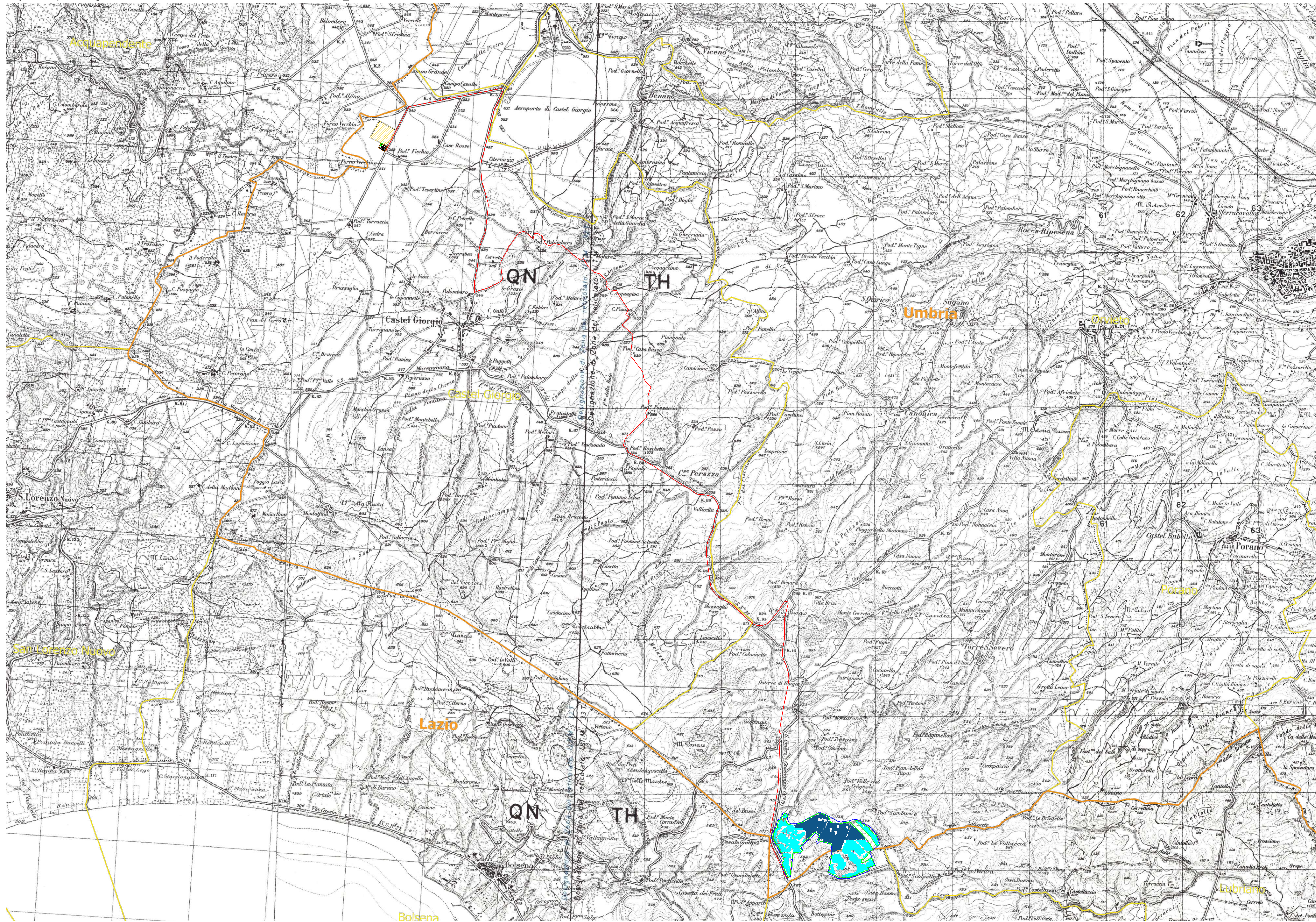
Layout impianto agrivoltaico e cavidotto fino alla sottostazione su IGM, scala 1:25000
