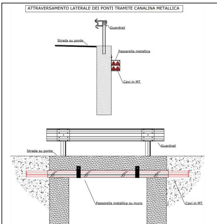
Figura 2: Attraversamento con posa cavidotto entro una canalina metallica al lato del ponte
