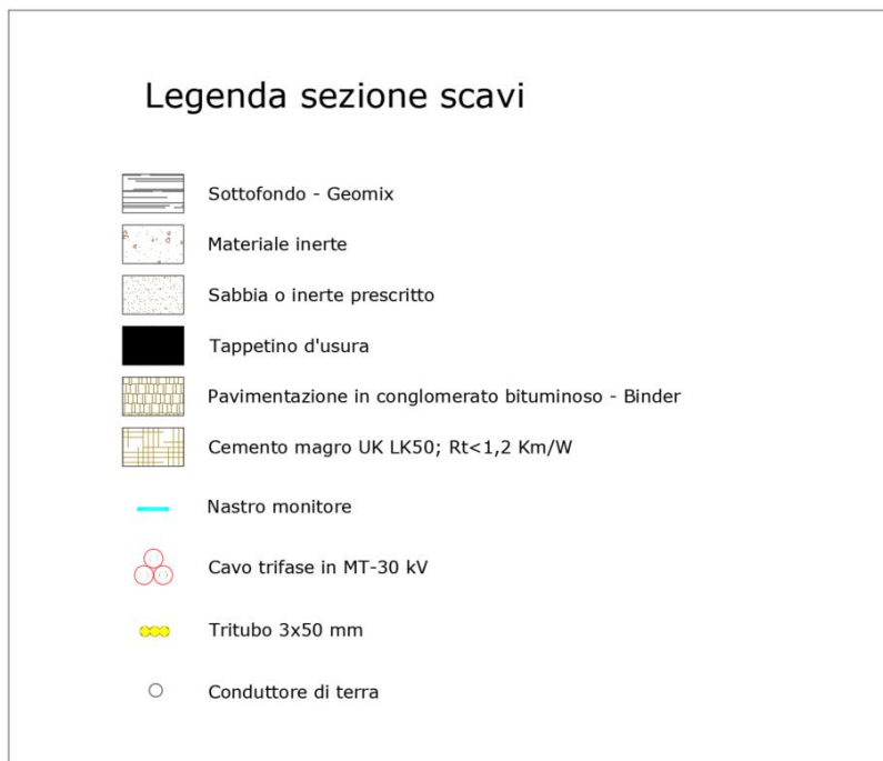
Figura 8: Materiali di riempimento per tipologia di scavo
