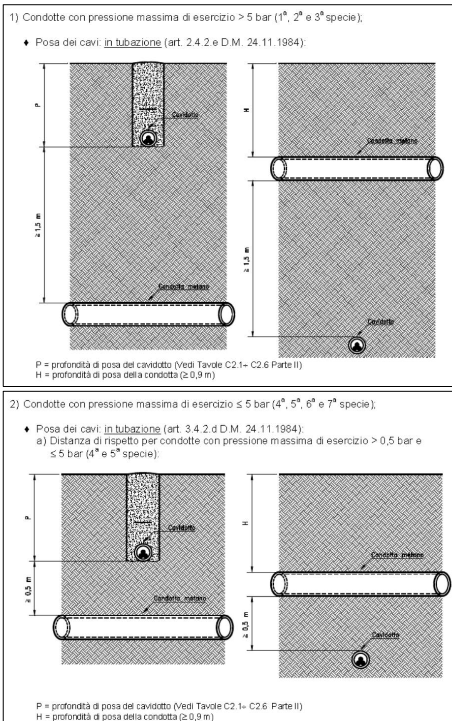
Figura 3: Tipico attraversamento di un gasdotto interrato
