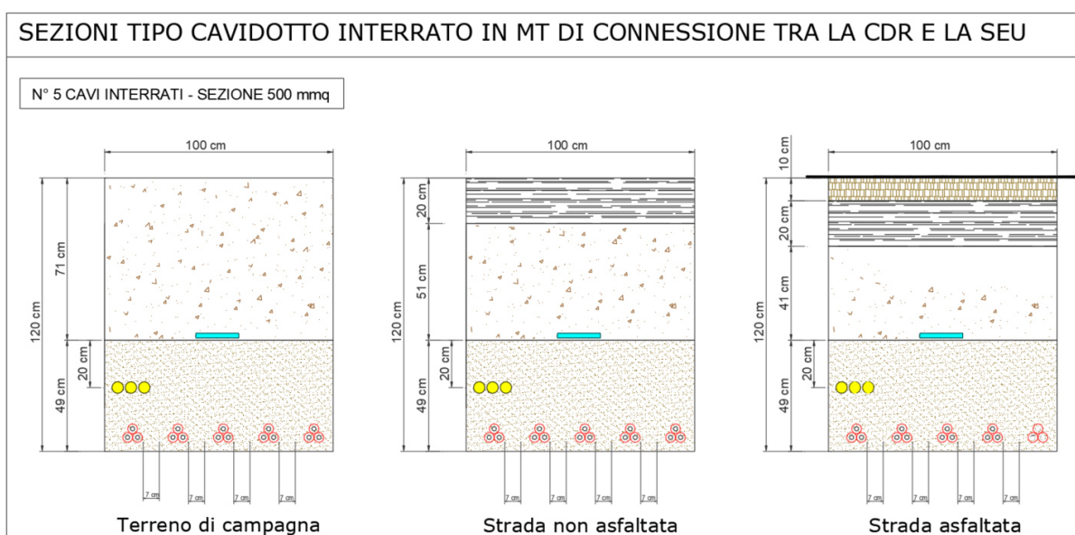
Figura 7: Sezioni degli scavi in MT
