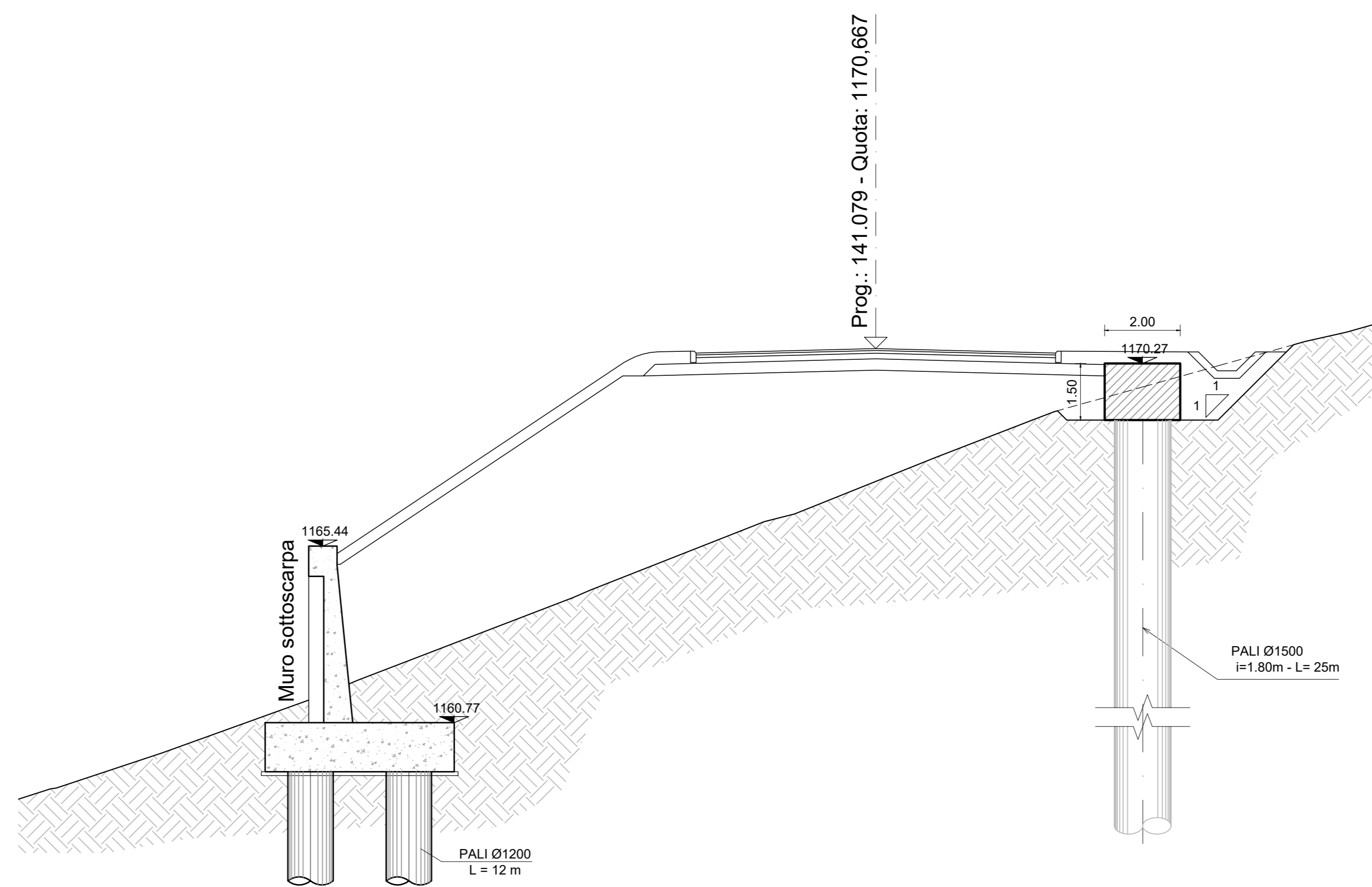
SEZIONE Prog. 141+079 Scala 1:100
