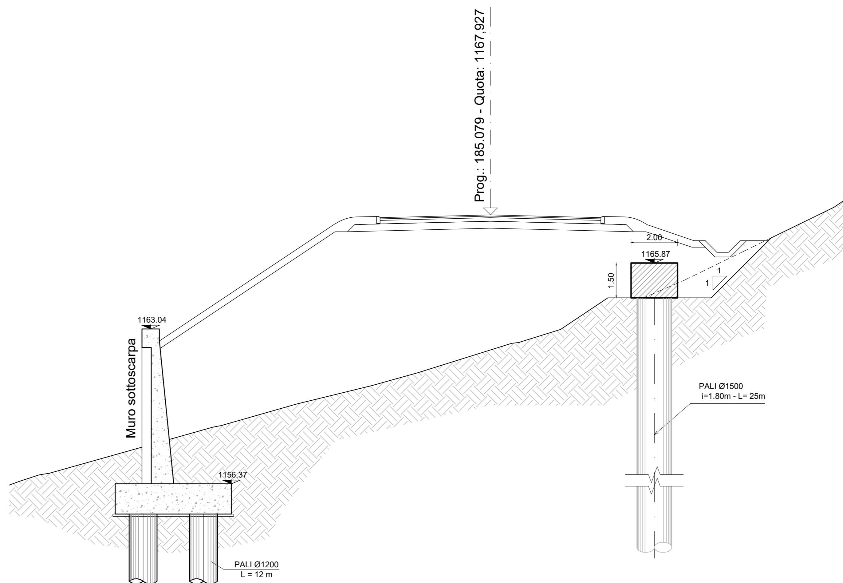
SEZIONE Prog. 185.079 Scala 1:100
