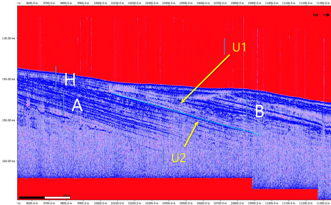
Figura 4-8 – Unità sismostratigrafica A e B. Zona di erosione di Unità B e relazione stratigrafica tra le unità.
