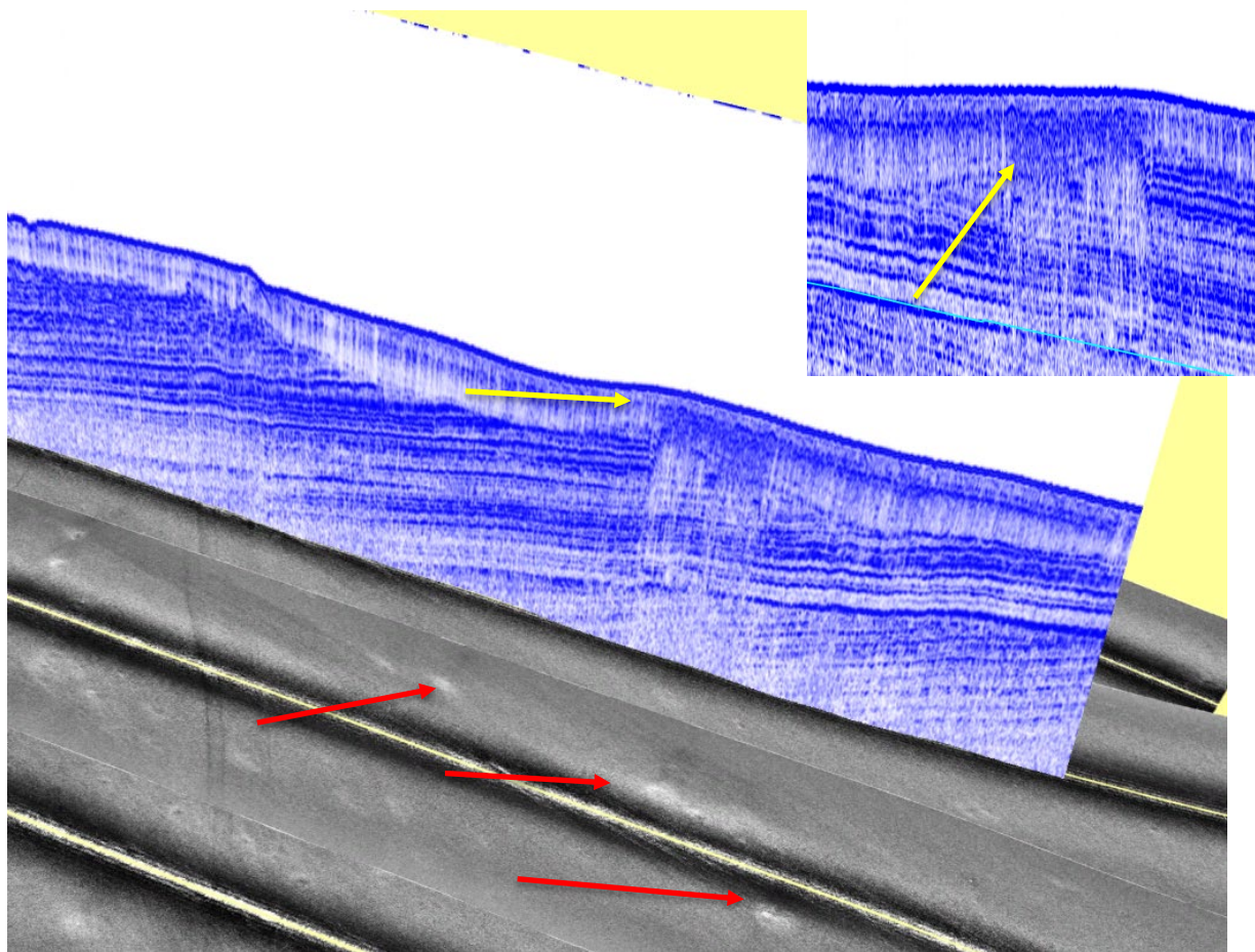
Figura 4-3 – Vista 3D Pale 04 A su mosaico dati SSS. Le frecce indicano le forme superficiali ascrivibili alle esalazioni gassose identificate nei dati SBP.
