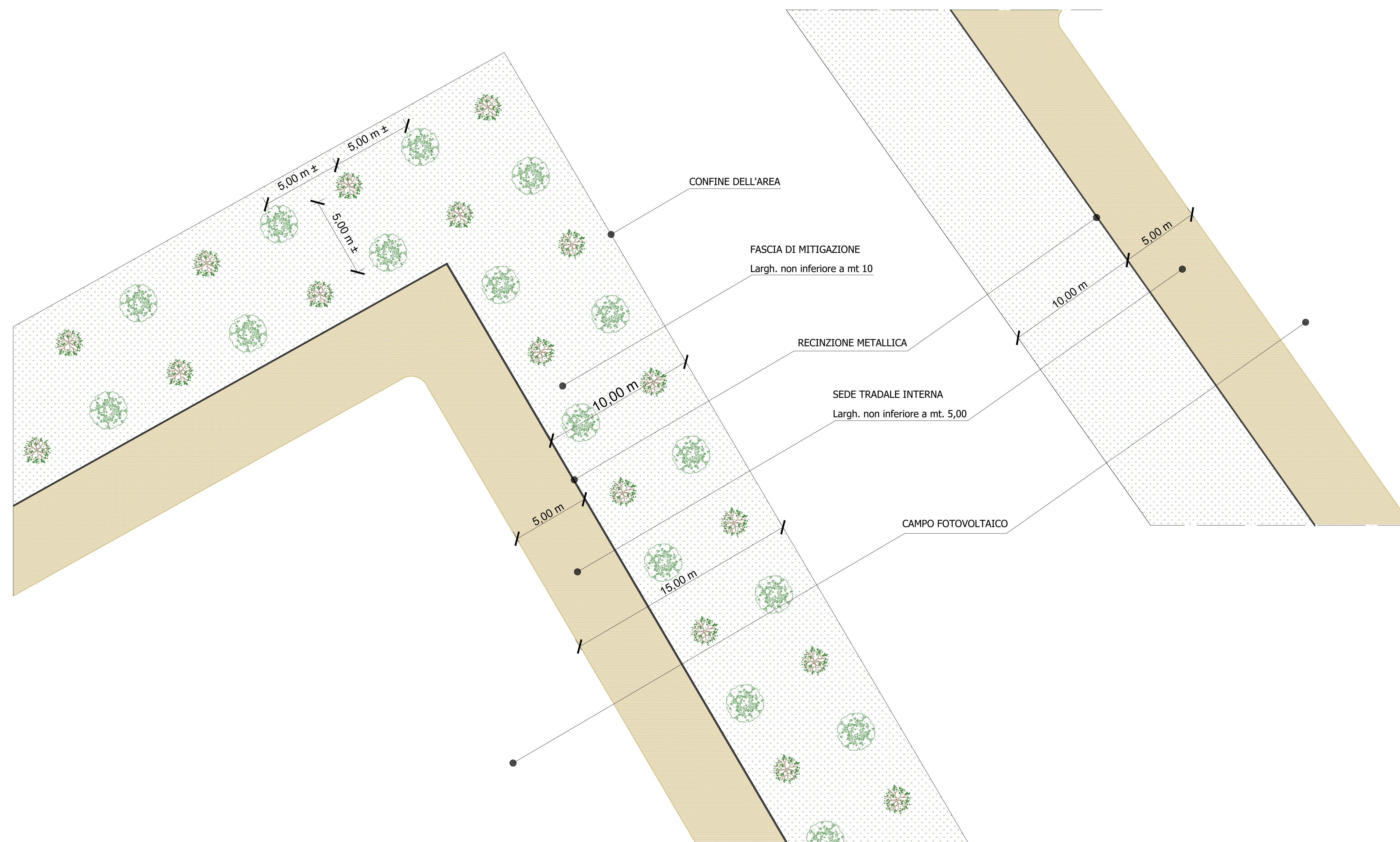
Fasce perimetrali di mitigazione: Stralcio pianta con dimensioni delle fasce - Scala 1:200
