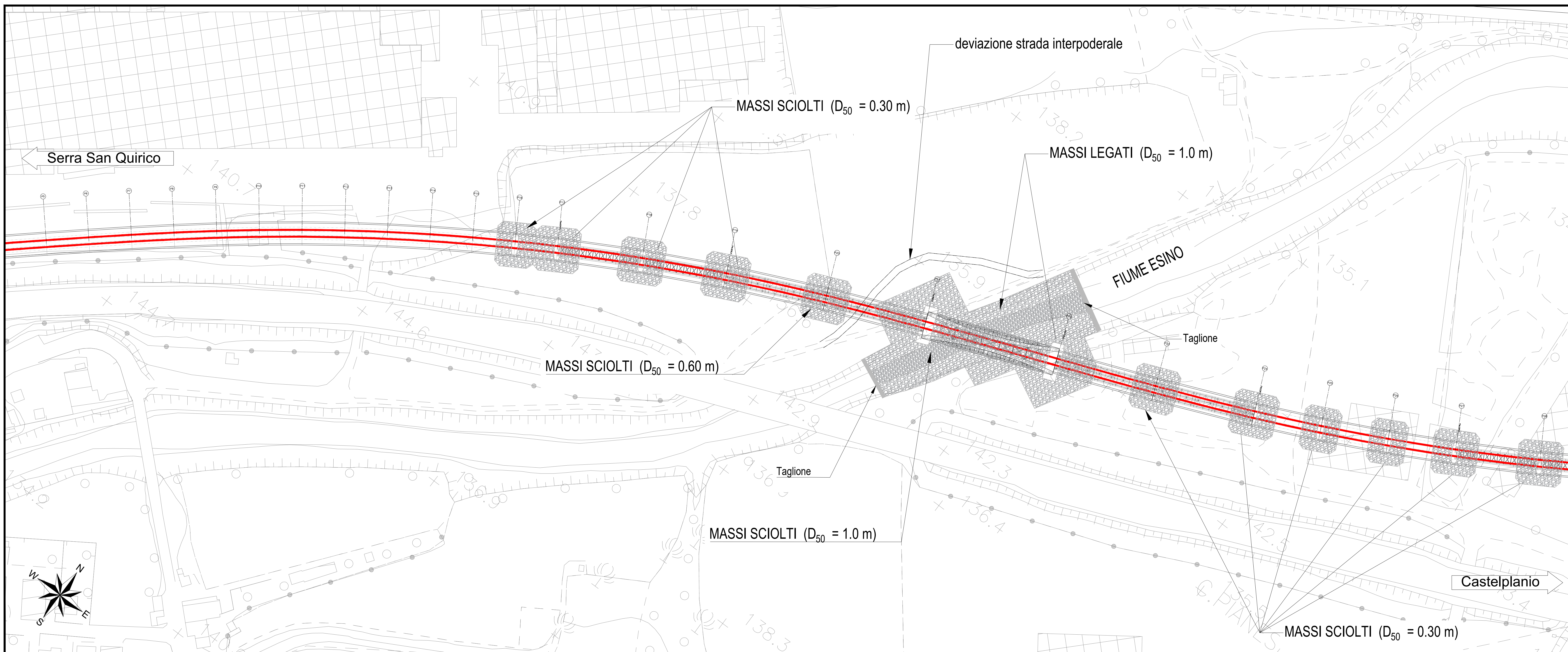
Pianta sistemazioni idrauliche - Fiume Esino - scala 1:1000
