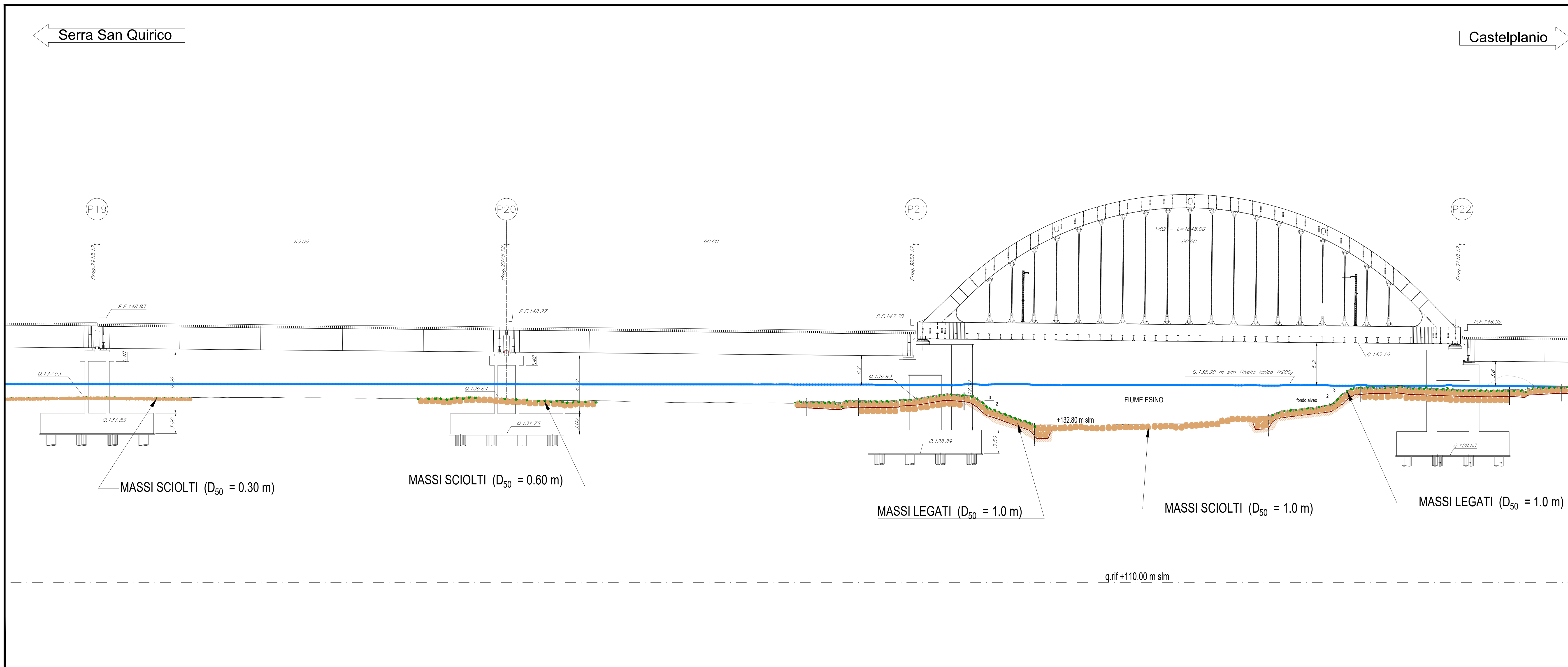
Sezione sistemazioni idrauliche - Fiume Esino - scala 1:250
