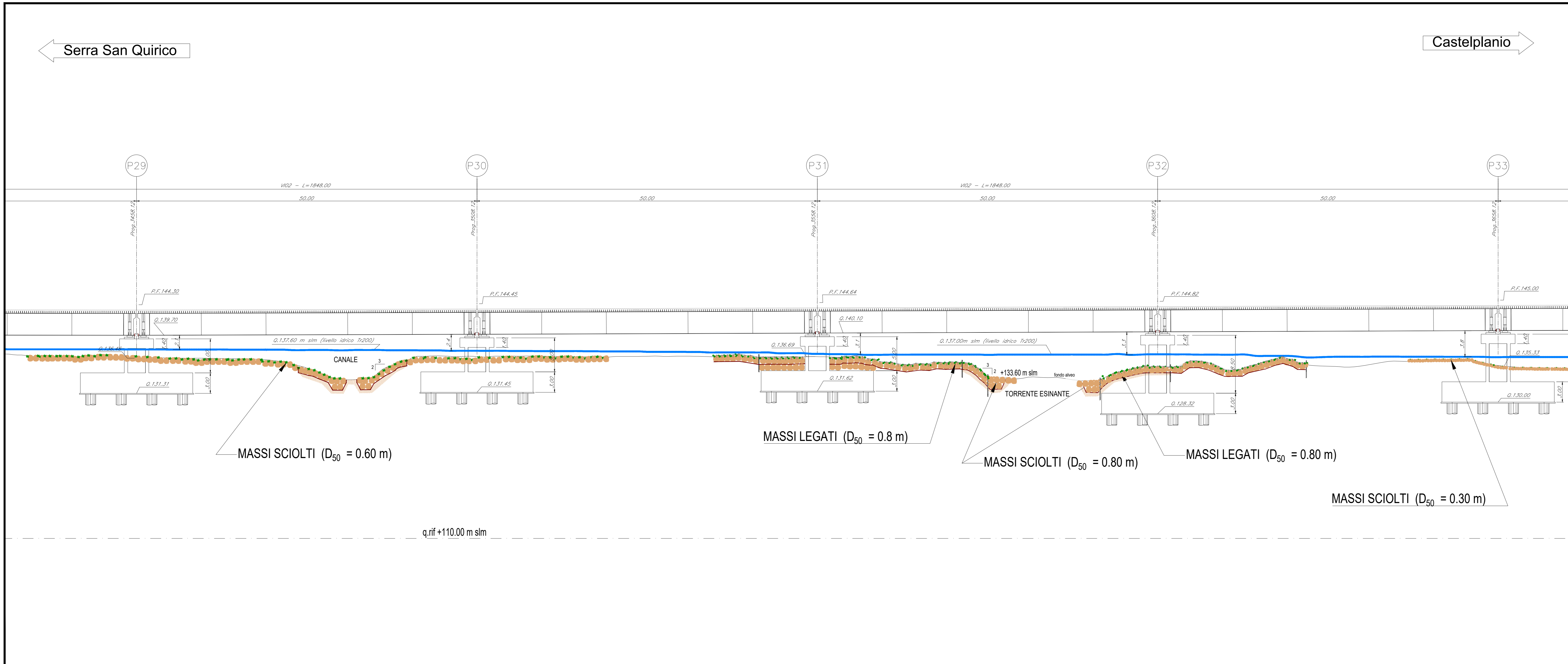
Sezione sistemazioni idrauliche - Fiume Esino (T. Esinante) - scala 1:250
