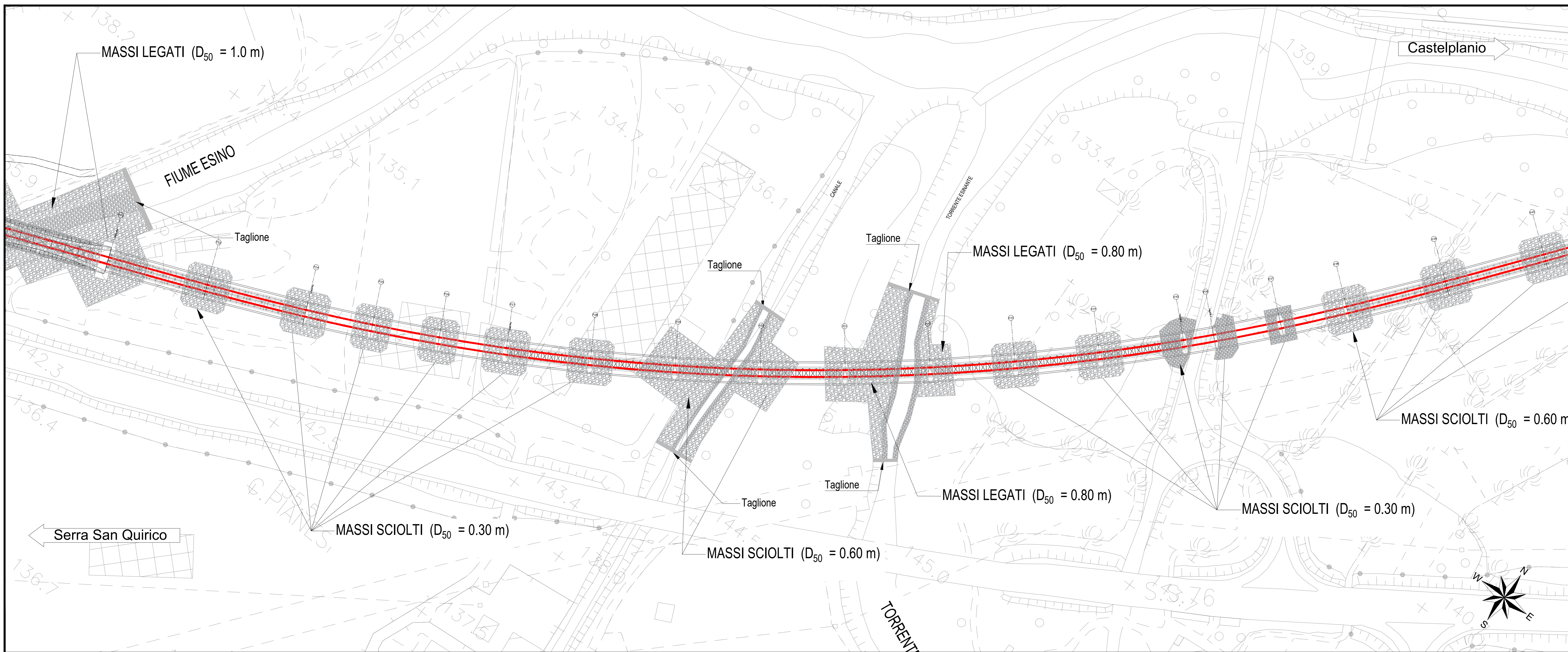
Pianta sistemazioni idrauliche - Fiume Esino (T. Esinante) - scala 1:1000
