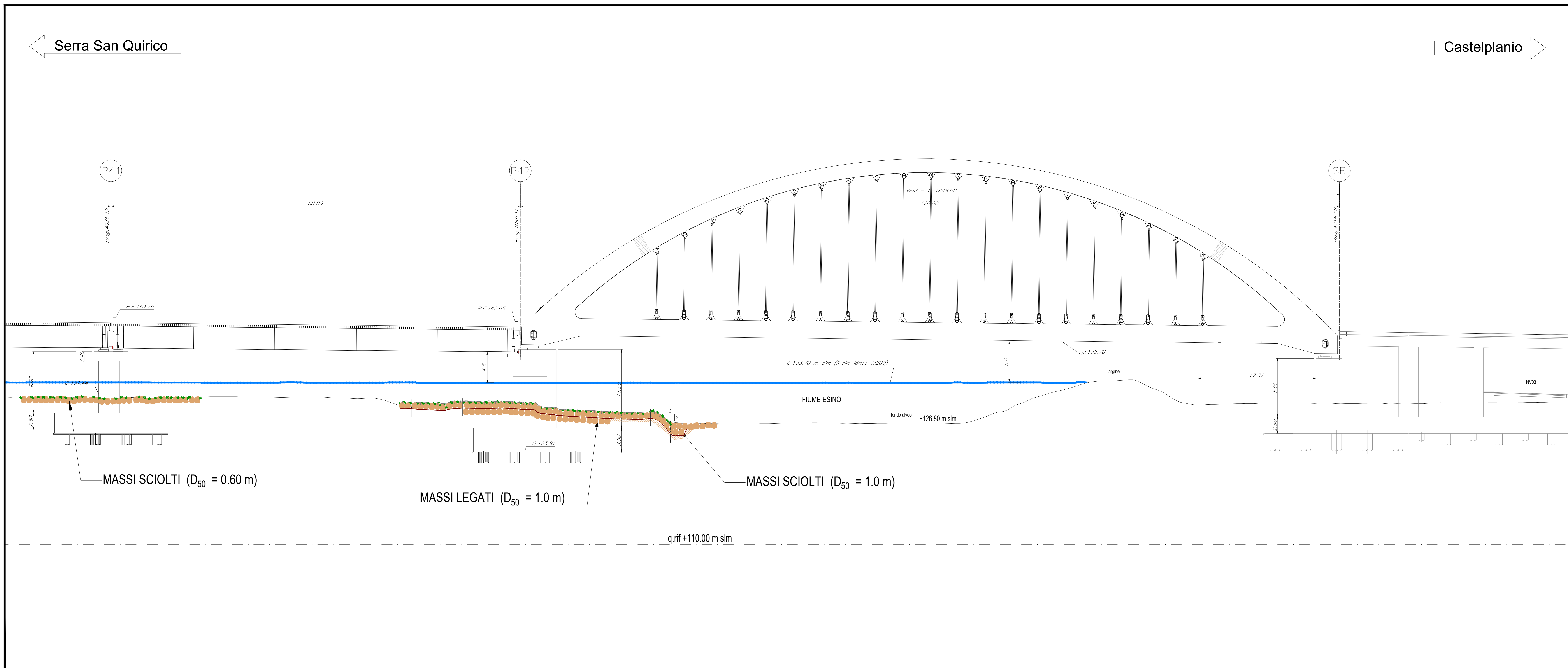
Sezione sistemazioni idrauliche - Fiume Esino - scala 1:500
