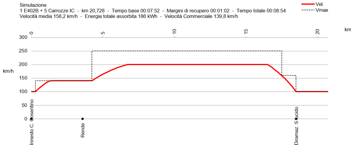
Figura 14: Diagramma di velocità E402B+5 carrozze IC (diramaz. S.Lucido)
