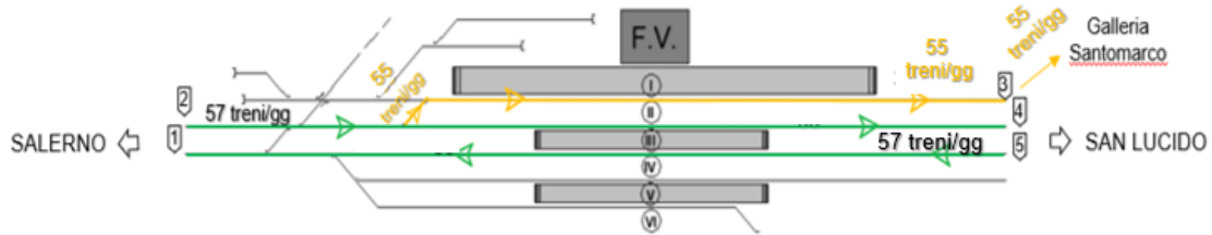
Figura 19: Layout Paola (radice lato Salerno)
