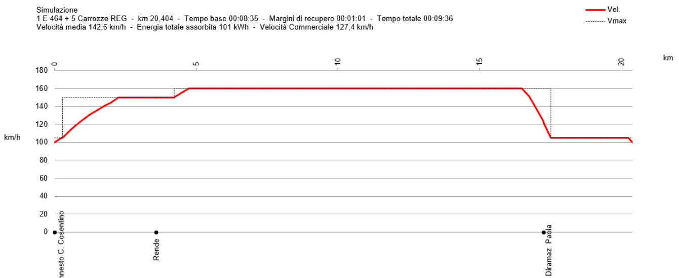
Figura 11: Diagramma di velocità E464+5 carrozze REG (diramaz. Paola)
