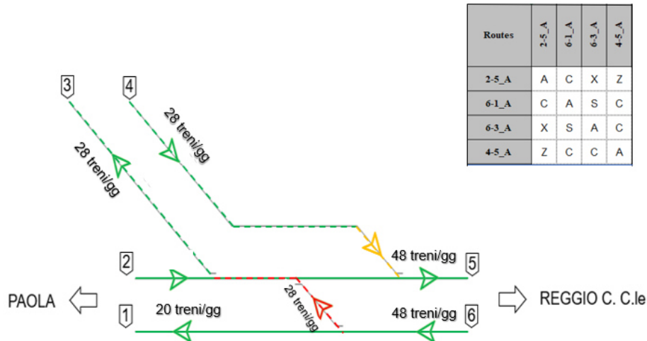
Figura 15: Layout collegamento Cosenza-S.lucido in deviato
