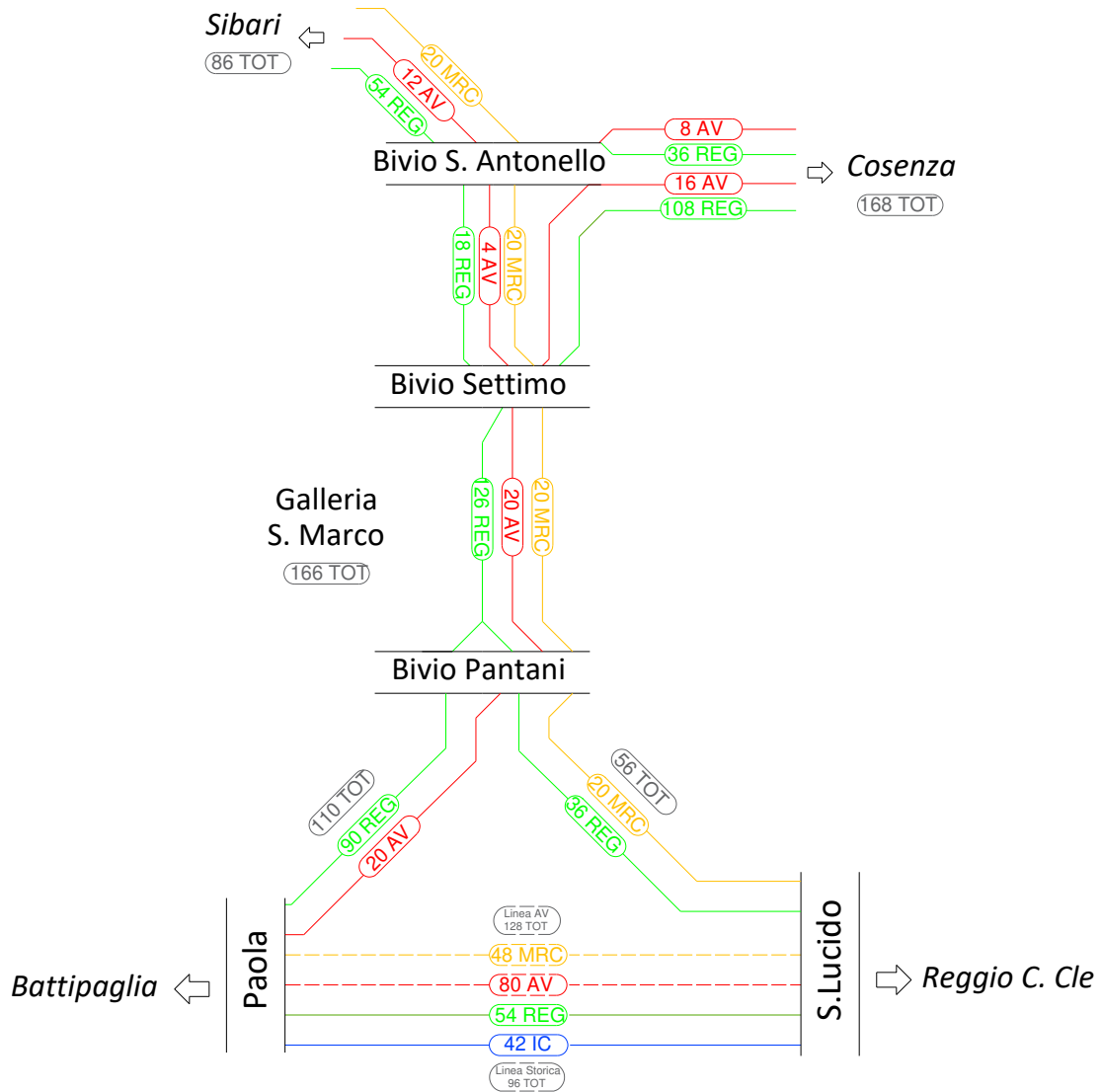
Figura 8: Modello di esercizio futuro (scenario di regime)
