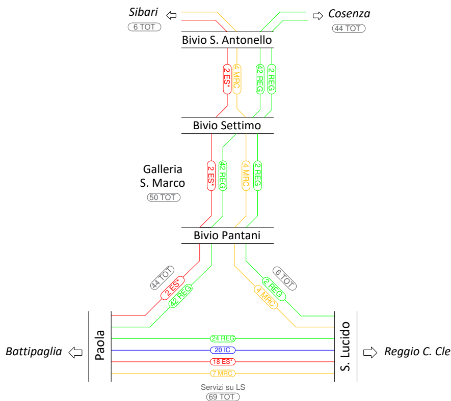
Figura 5: Modello di esercizio attuale
