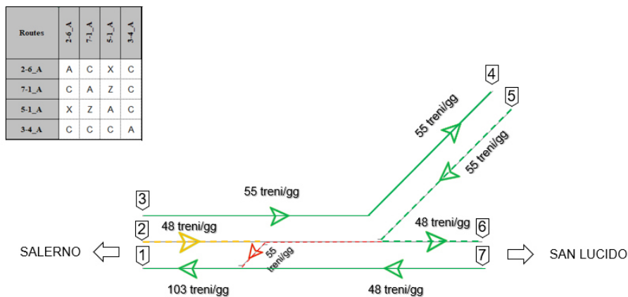
Figura 17: Layout diramazione Paola (diramazione lato S.Lucido)
