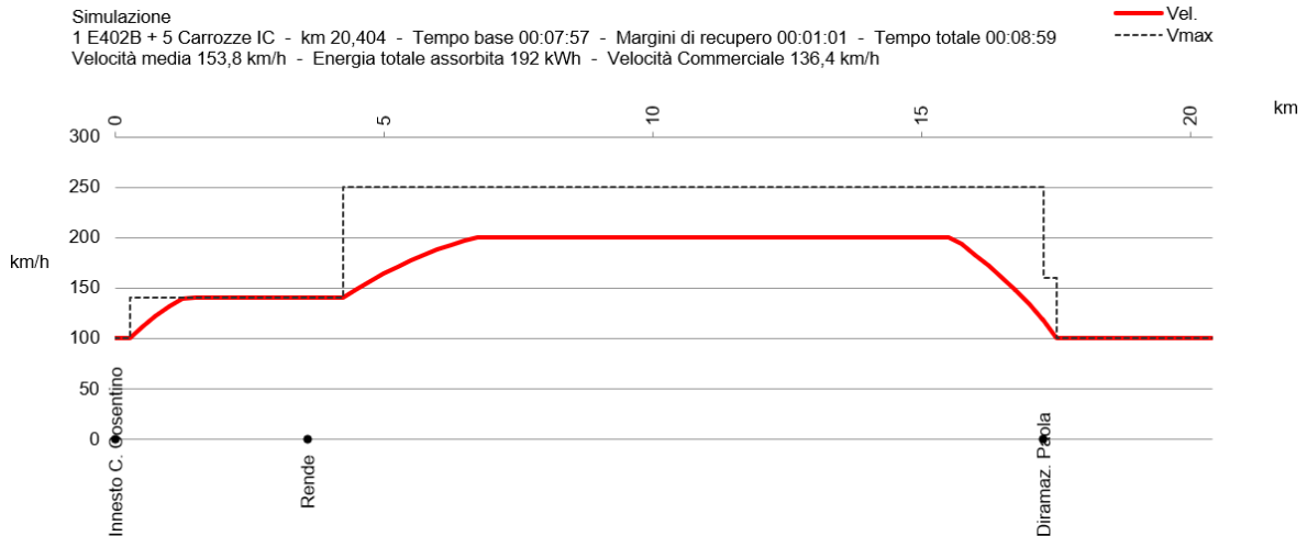
Figura 12: Diagramma di velocità E402B+5 carrozze IC (diramaz. Paola)
