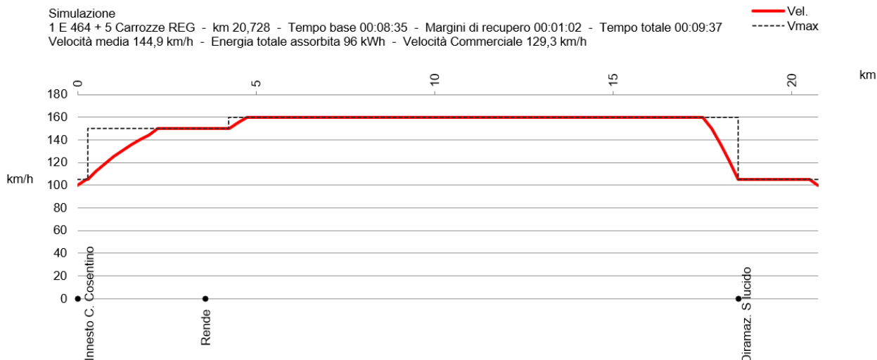
Figura 13: Diagramma di velocità E464+5 carrozze REG (diramaz. S.Lucido)
