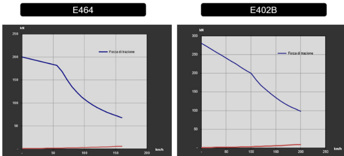
Figura 10: Curva di trazione
