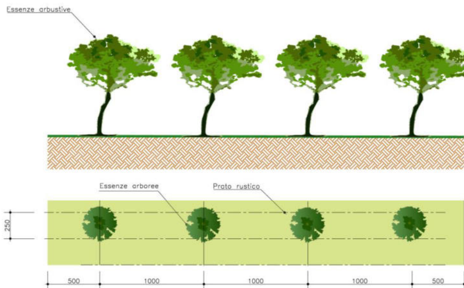
Figura 4-5 – MODULO E – Filare monospecie
