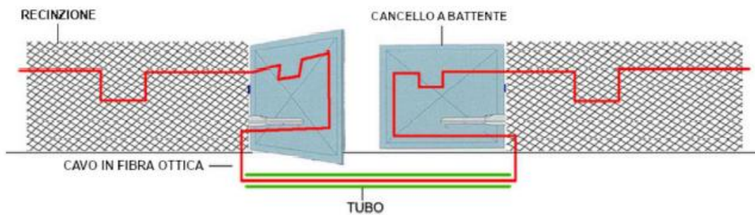
Schema di installazione cavo in fibra ottica su recinzione.
