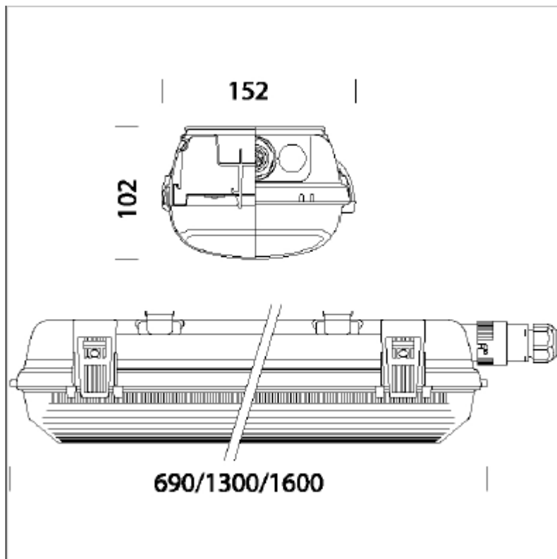
Plafoniera LED tipo ECHO.
