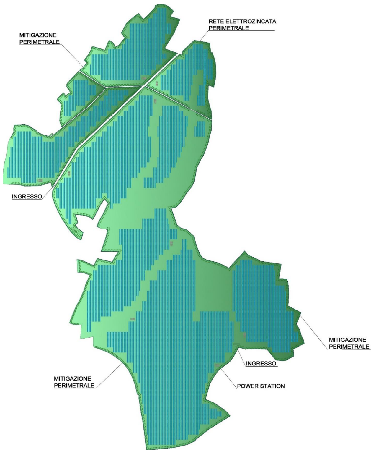
Figura 3-2 Layout corpo A
