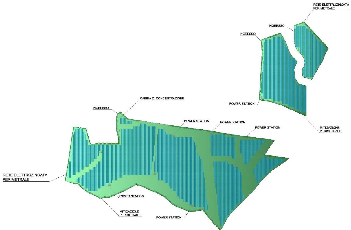
Figura 3-4 Layout corpo C e D
