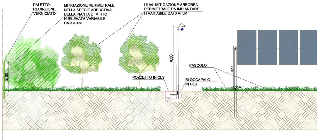
Figura 3-1 Dettaglio recinzione e mitigazione perimetrale
