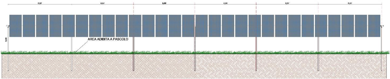
VISTA LATERALE CON ROTAZIONE DI 55° - SCALA 1:100
