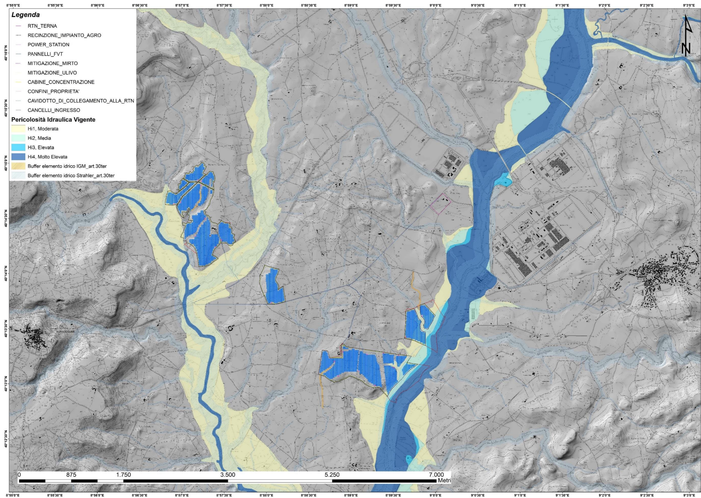
Figura 5-1 Inquadramento Pericolosità idraulica PGRA 2021(Hi)
