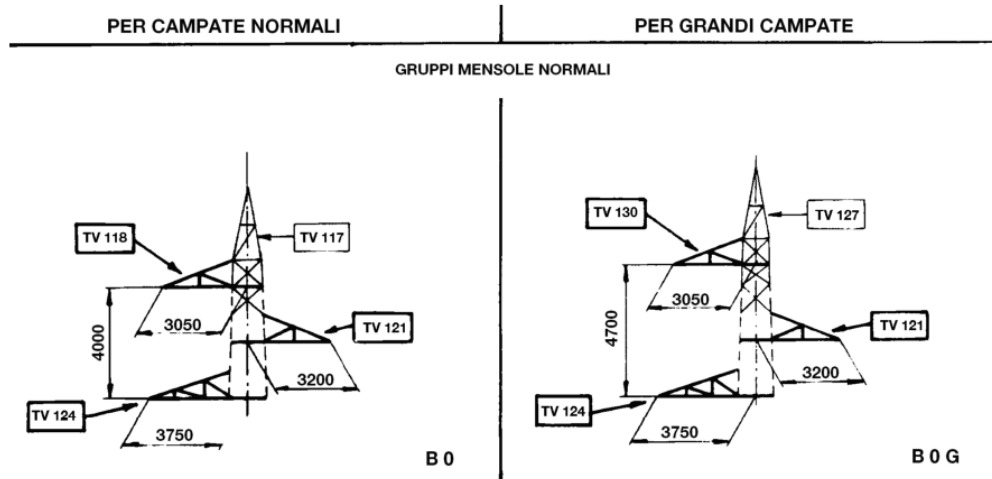
Fig. 4: geometria dei conduttori sostegno in semplice terna a 150kV - Tipo P e V
