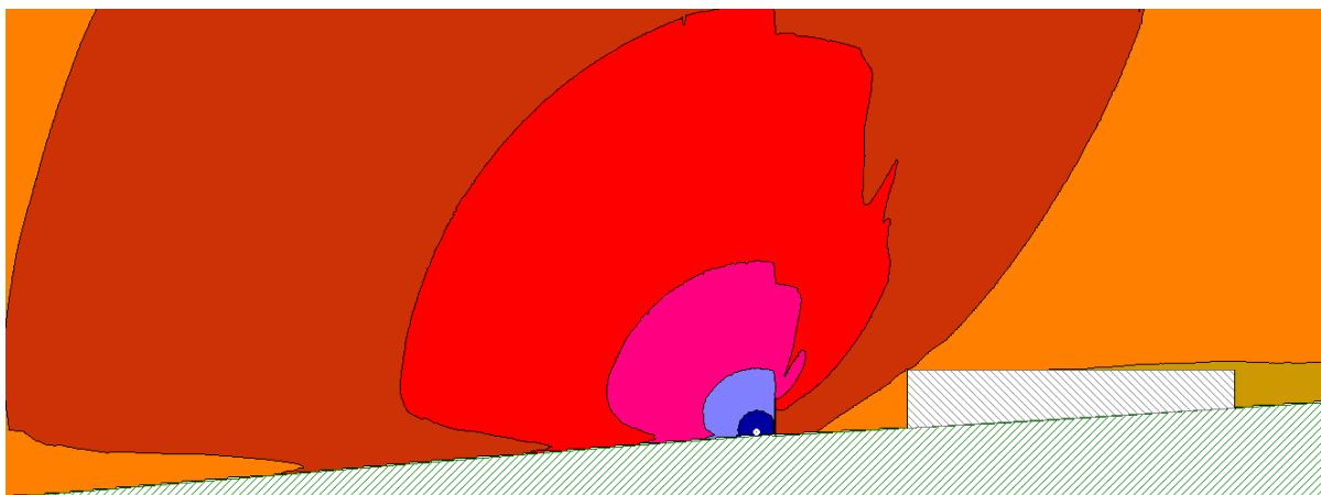
Figura 5 Rumore generato dalla lavorazione di posa cavidotto dopo le opere di mitigazione riceettore RC03
