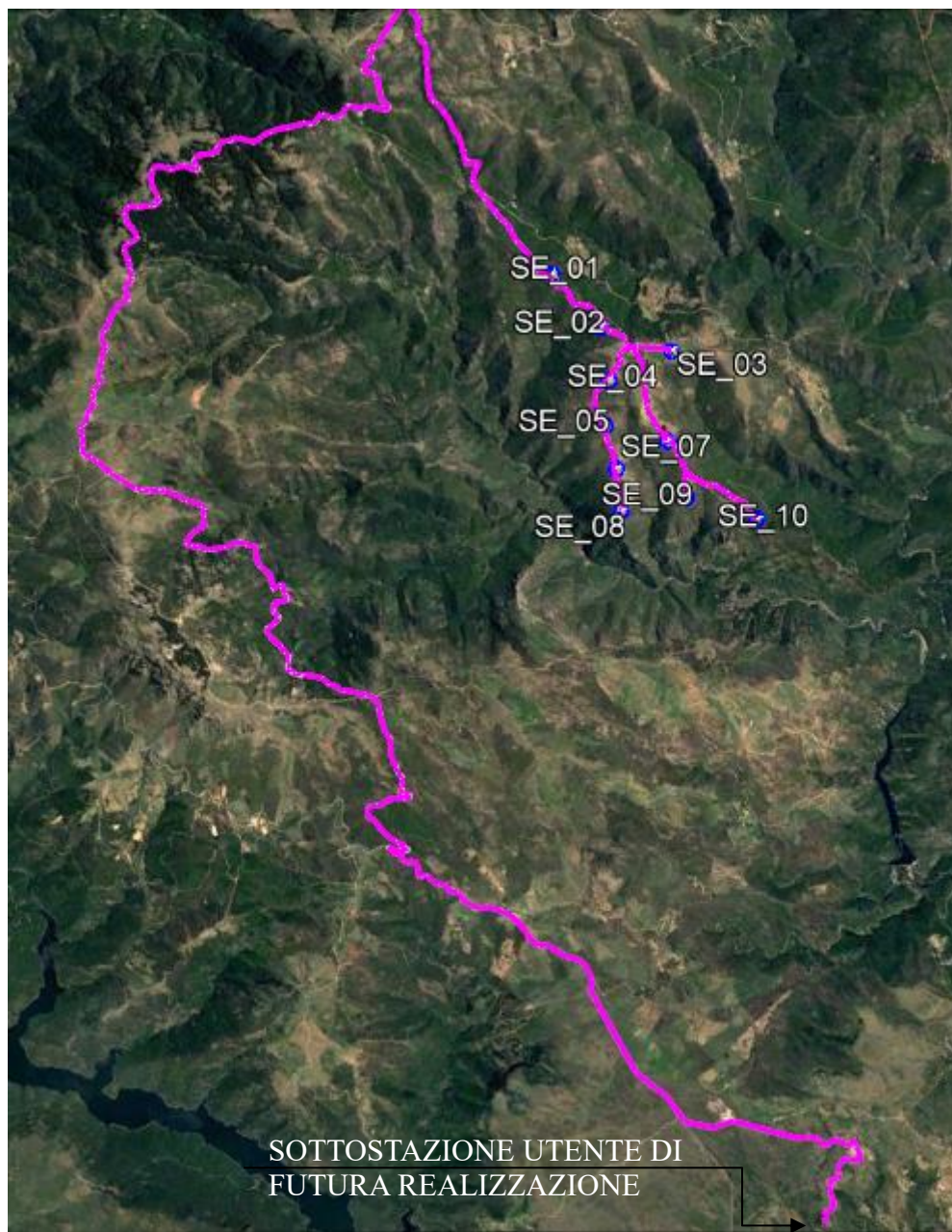
Figura 2 Area di ubicazione del parco eolico e della connessione alla Sottostazione Utente di futura realizzazione.
