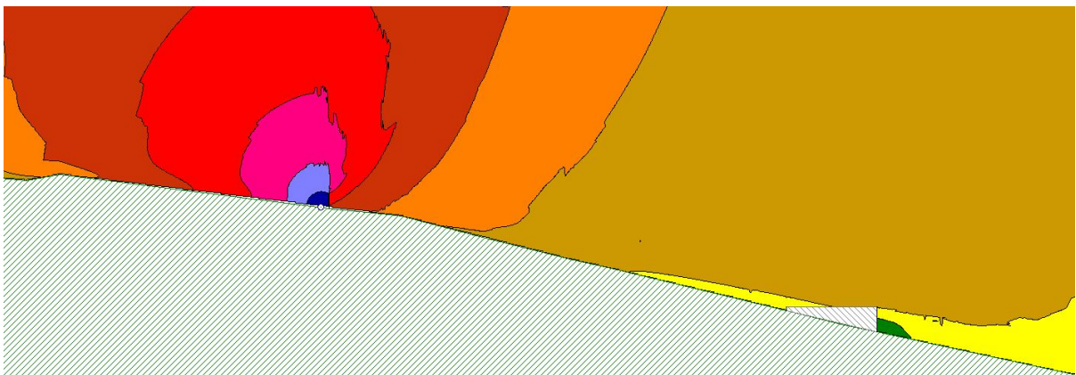
Figura 3 Rumore dalla lavorazione di posa cavidotto dopo le opere di mitigazione nel ricettore R04
