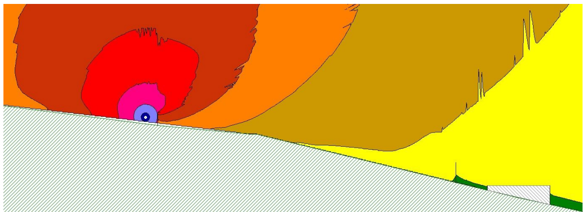
Figura 4 Rumore dalla lavorazione di adeguamento stradale dopo le opere di mitigazione nel ricettore R04
