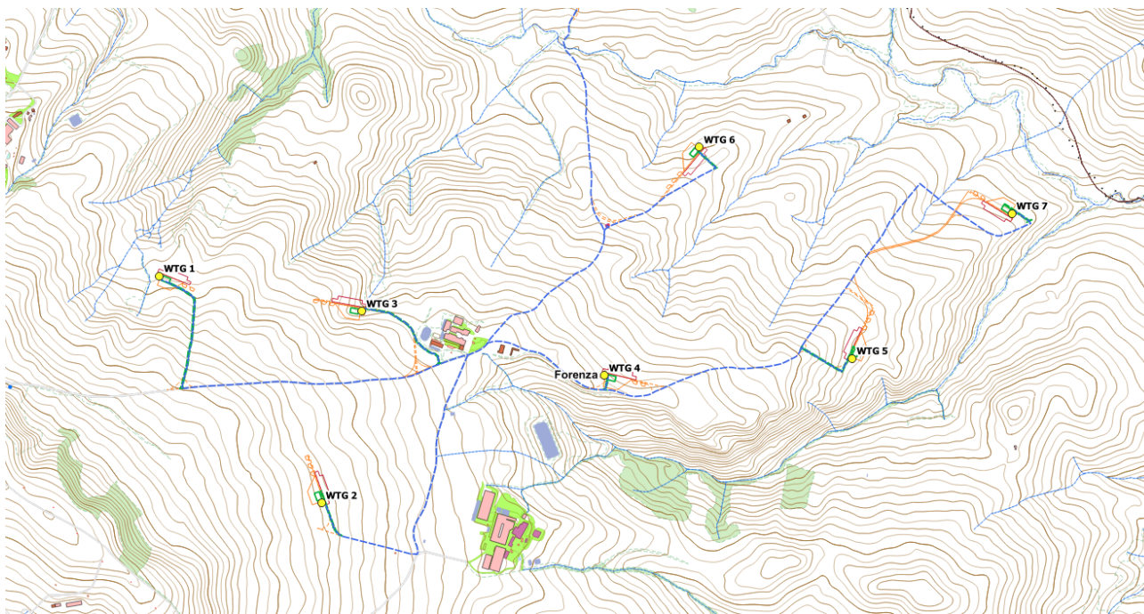
Figura 2.1-3: Area di sito su base CTR
