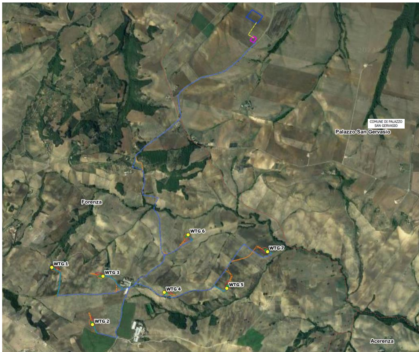
Figura 2.1-4: Area di sito: dettaglio layout di progetto su ortofoto
