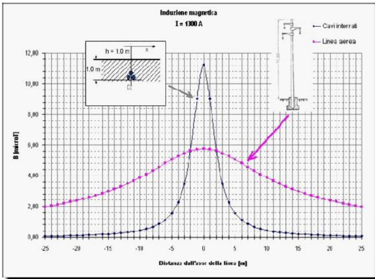
Attenuazione dell'induzione magnetica dovuta all'interramento dei cavi
