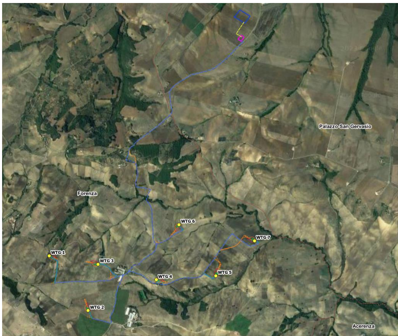
Figura 4-4: Area di intervento: dettaglio layout di progetto su ortofoto
