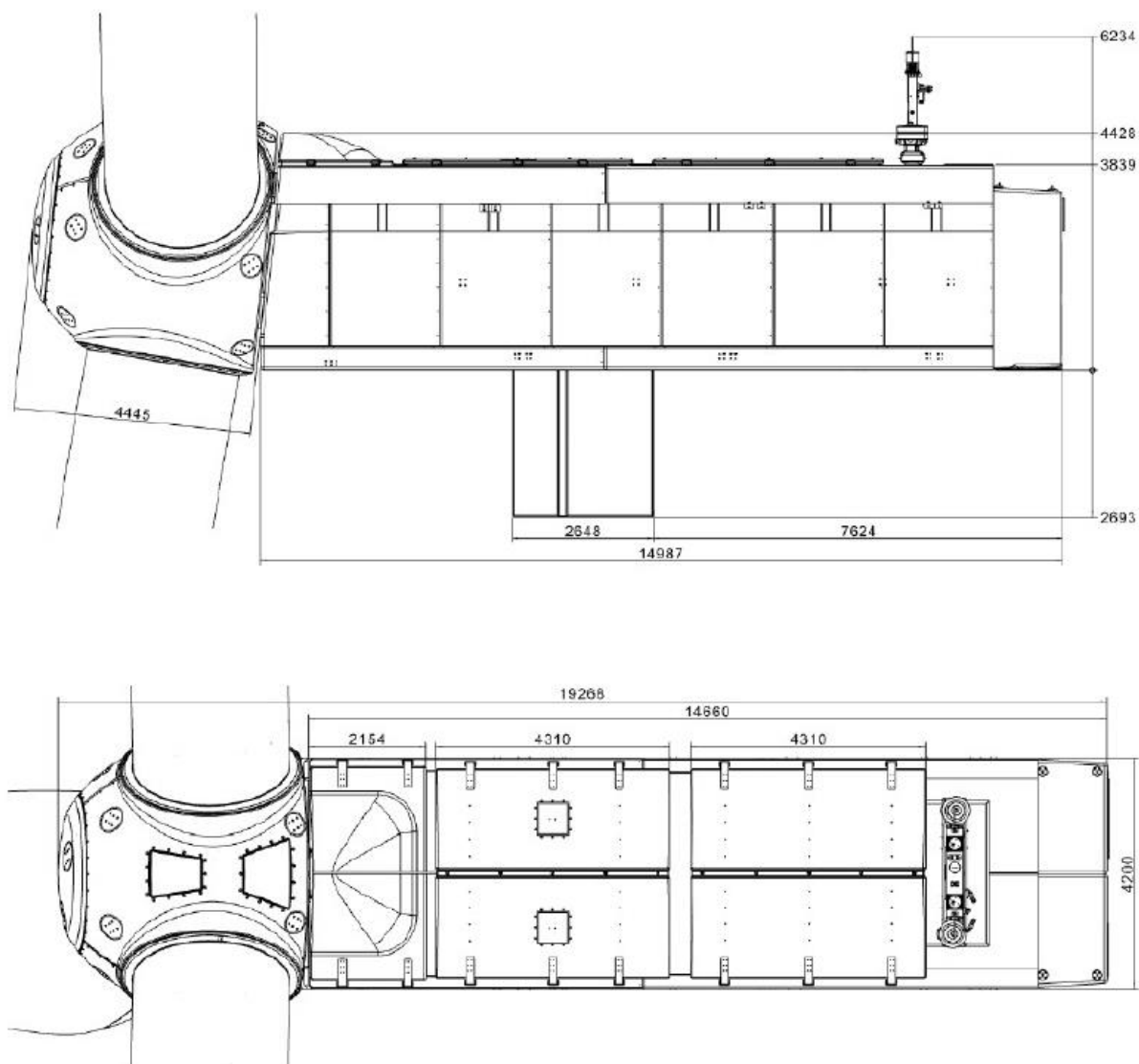
Figura c-2: Tipico navicella WTG
