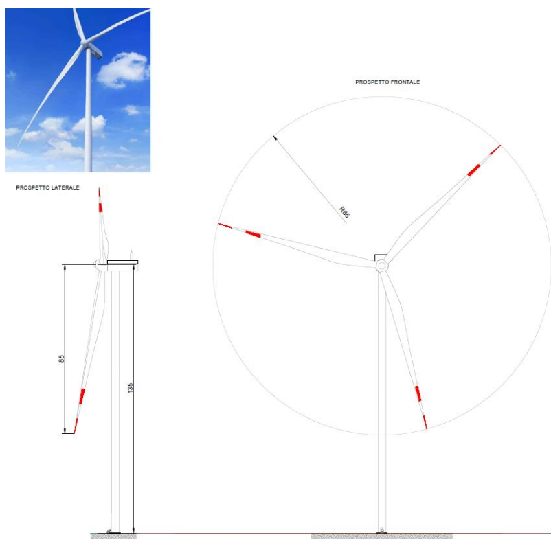
Figura c-1: Struttura aerogeneratore
