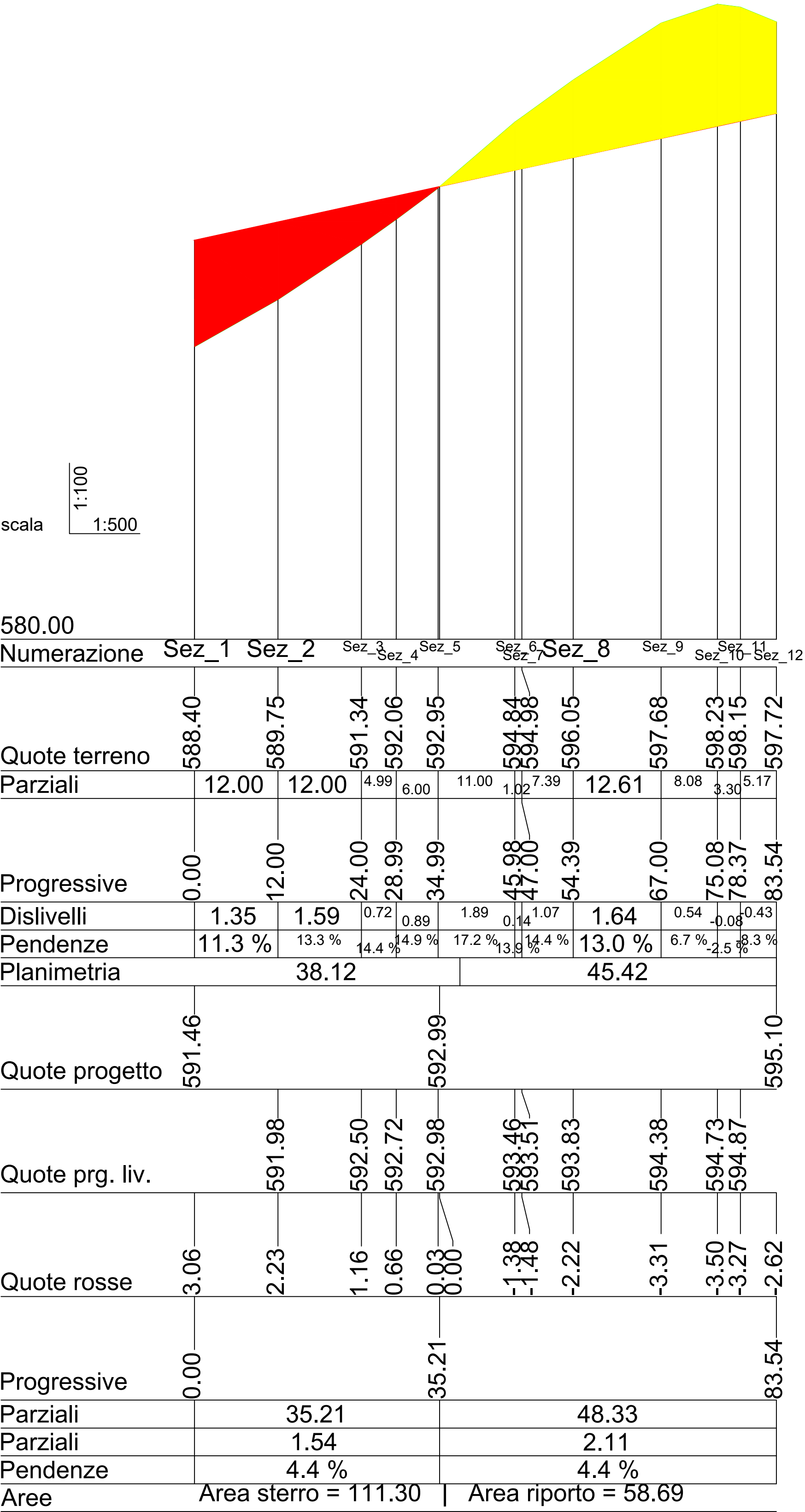
Profilo PROGETTO - WTG 4
