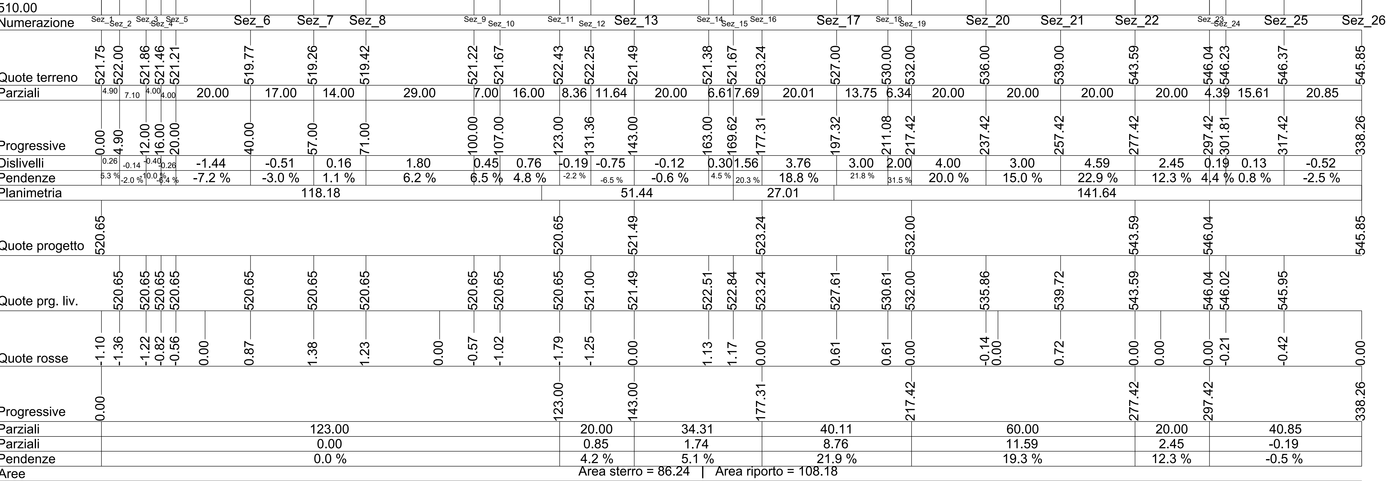
Profilo PROGETTO - WTG 5
