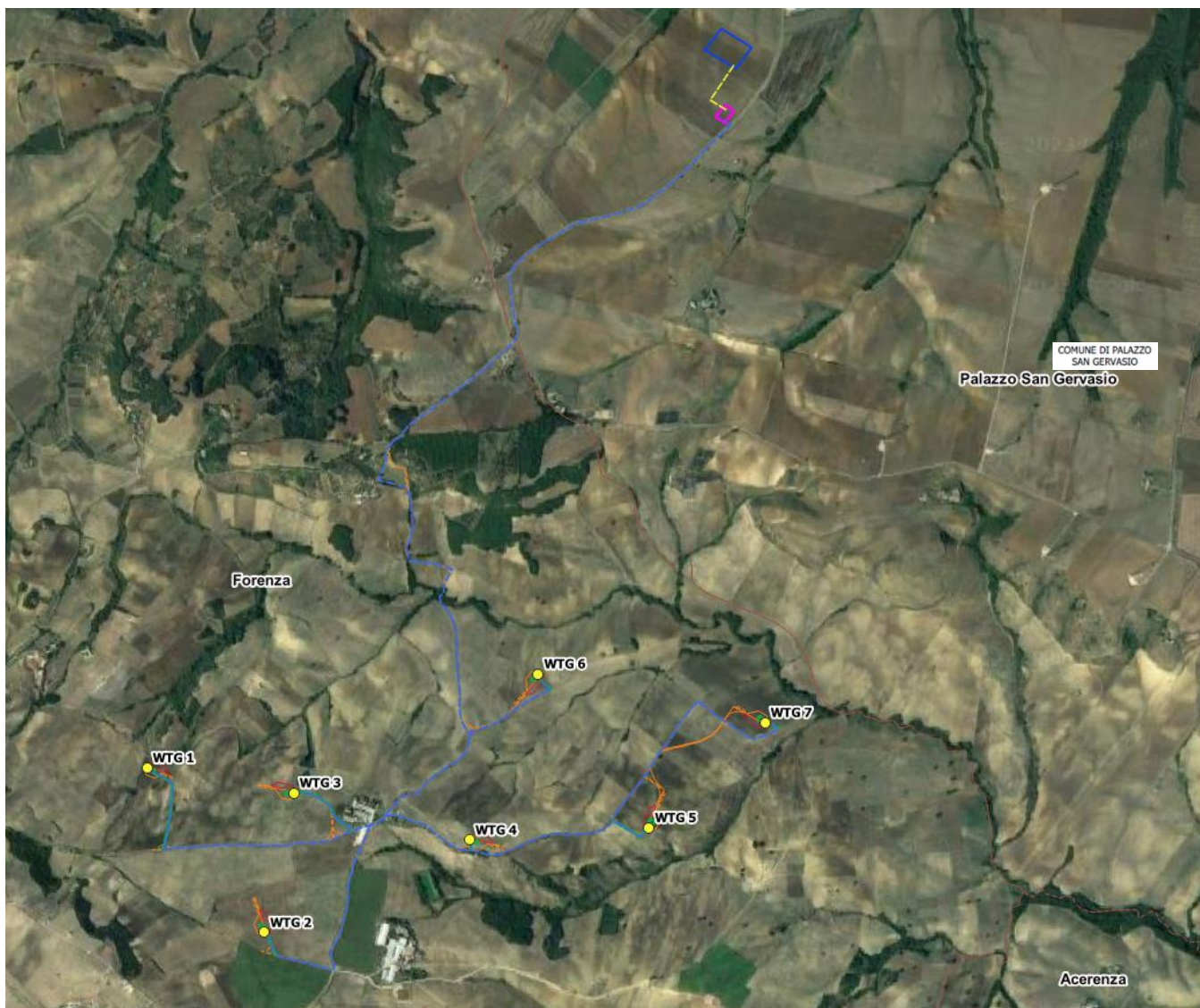
Figura 2-4: Area di sito: dettaglio layout di progetto su ortofoto
