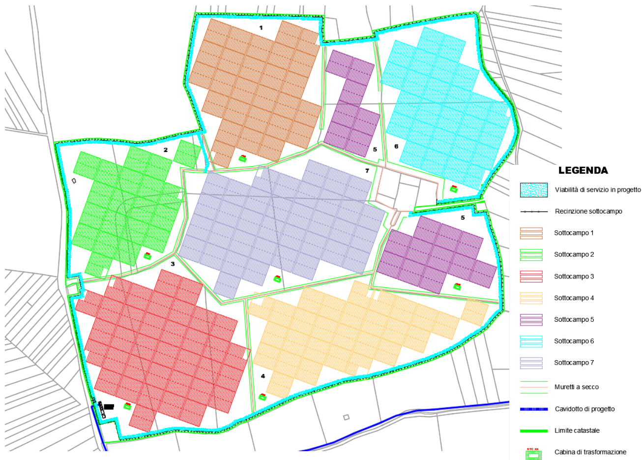
Figura 3.1 – Inquadramento area impianto e sottocampi
