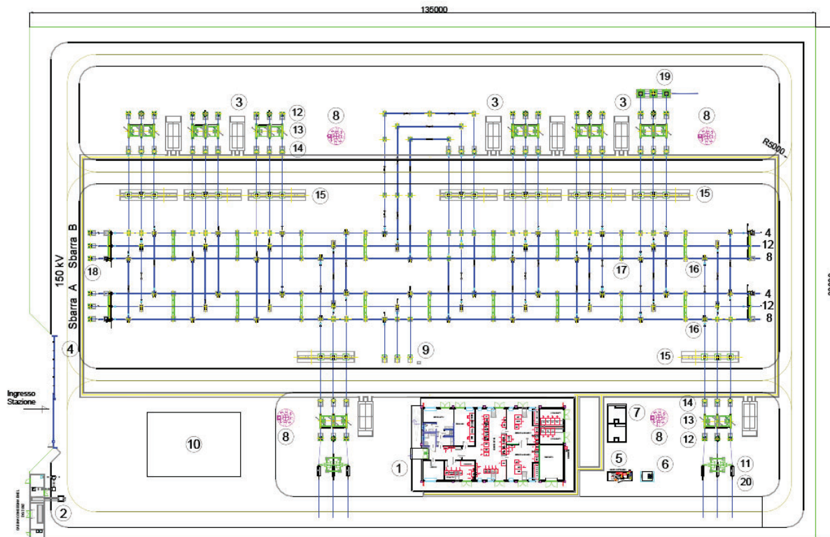
Figura 6-1: Planimetria nuova Stazione Elettrica 150 kV
