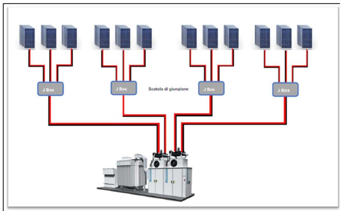
Tipico configurazione Stazione inverter centralizzata
