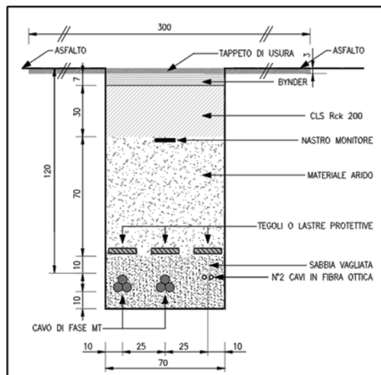
Tipico cavidotto su strada asfaltata
