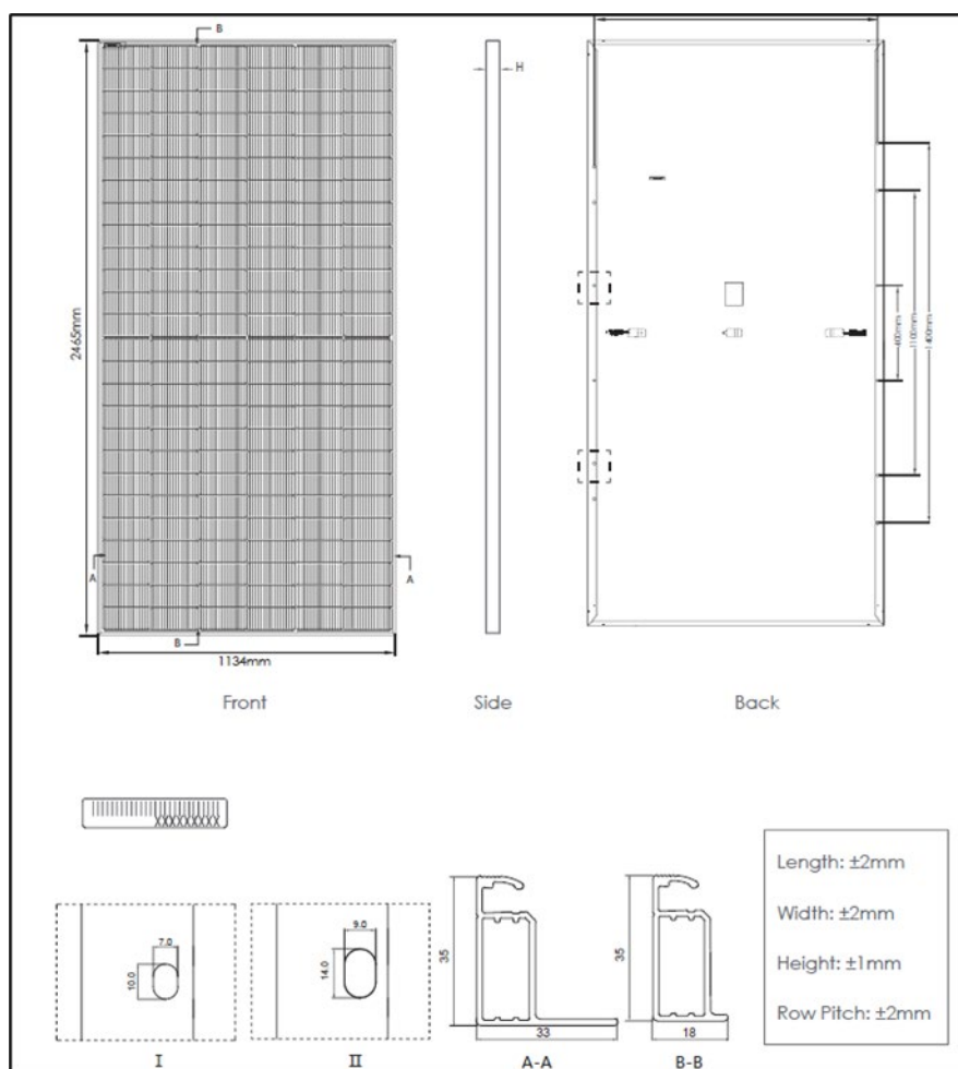
Dettaglio del Pannello Fotovoltaico (Vista frontale, posteriore e dimensioni)
