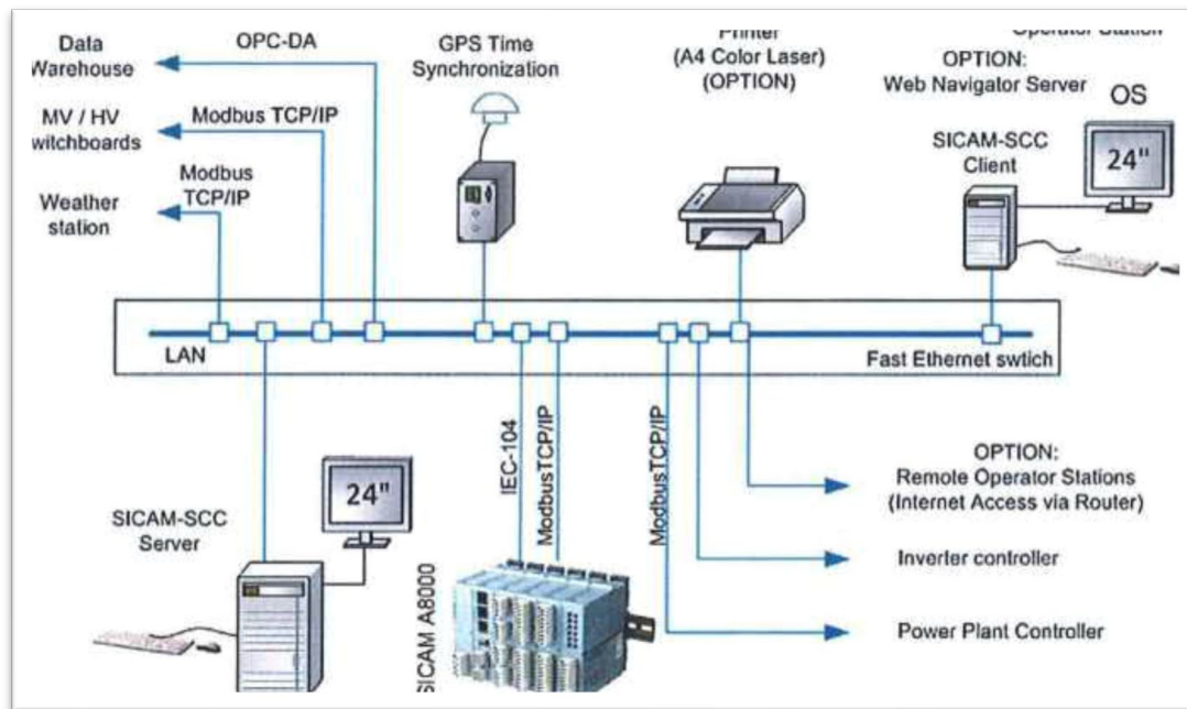
Layout di comunicazione
