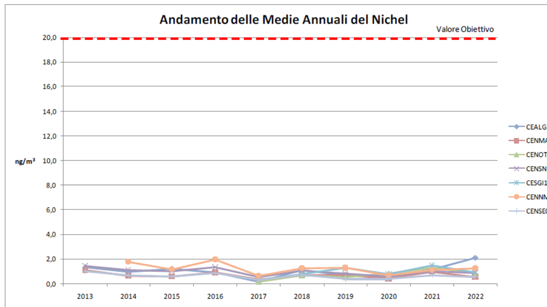
Figura 4-23: Grafico degli andamenti annuali del nichel nella Zona Rurale
