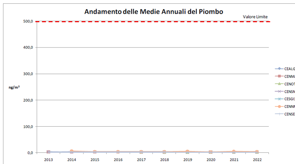
Figura 4-24: Grafico degli andamenti annuali del piombo nella Zona Rurale
