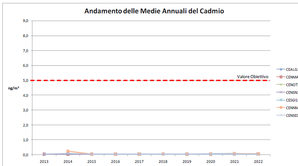
Figura 4-22: Grafico degli andamenti annuali del cadmio nella Zona Rurale
