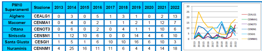
Figura 4-20: Superamenti di PM10 - Zona Rurale
