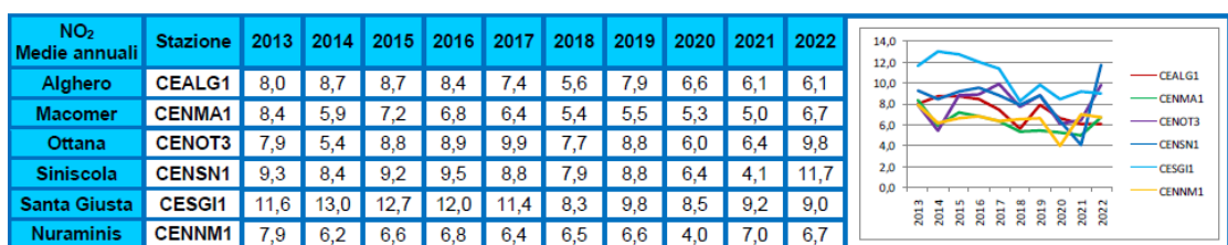
Figura 4-18: Medie annuali di biossido di azoto (µg/m 3 ) - Zona Rurale
