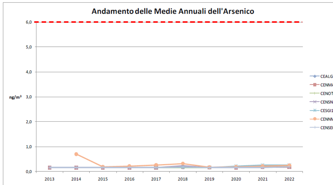
Figura 4-21: Grafico degli andamenti annuali dell'arsenico nella Zona Rurale
