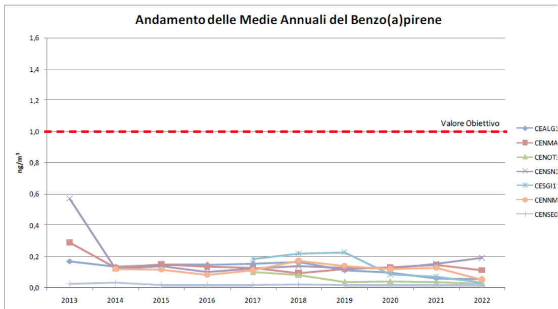
Figura 4-25: Grafico degli andamenti annuali del benzo(a)pirene nella Zona Rurale
