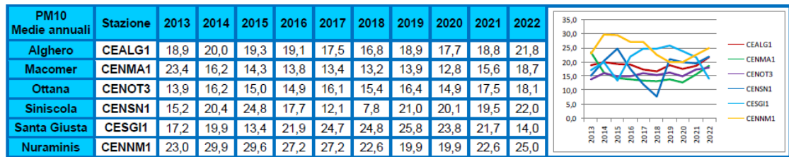
Figura 4-19: Medie annuali di PM10 ( \mu\text{g}/\text{m}^3 ) - Zona Rurale
