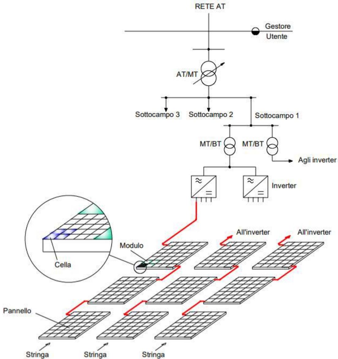
Immagine 4.6.1 Schema di impianto fotovoltaico.
