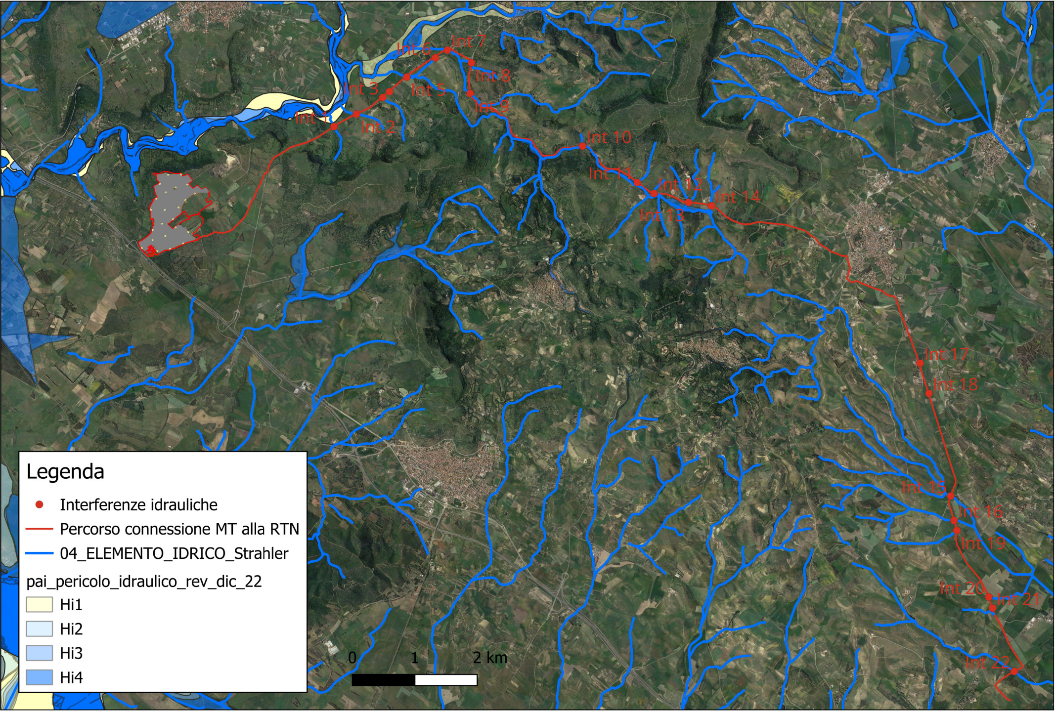
Planimetria inquadramento impianto e cavidotto MT su ortofoto - Scala 1:60.000
