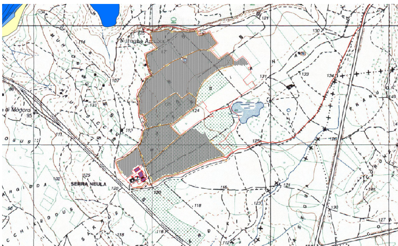
Figura 5: Planimetria di progetto su IGM con individuazione del reticolo idrografico della Regione Sardegna
