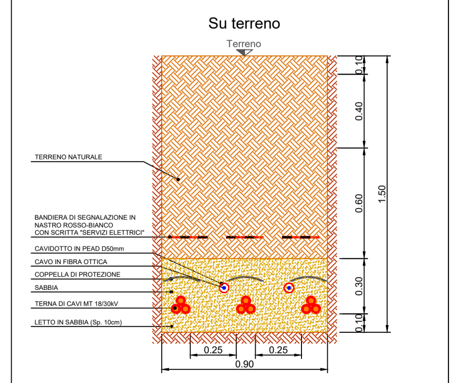
Tipologia E - Scavo a trincea su terreno - tre terne
