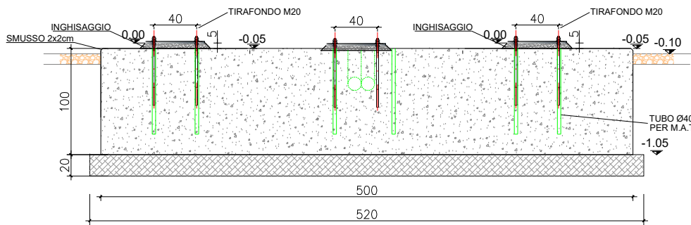
SEZIONE C-C
