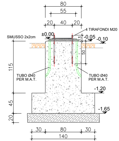
SEZIONE B-B
