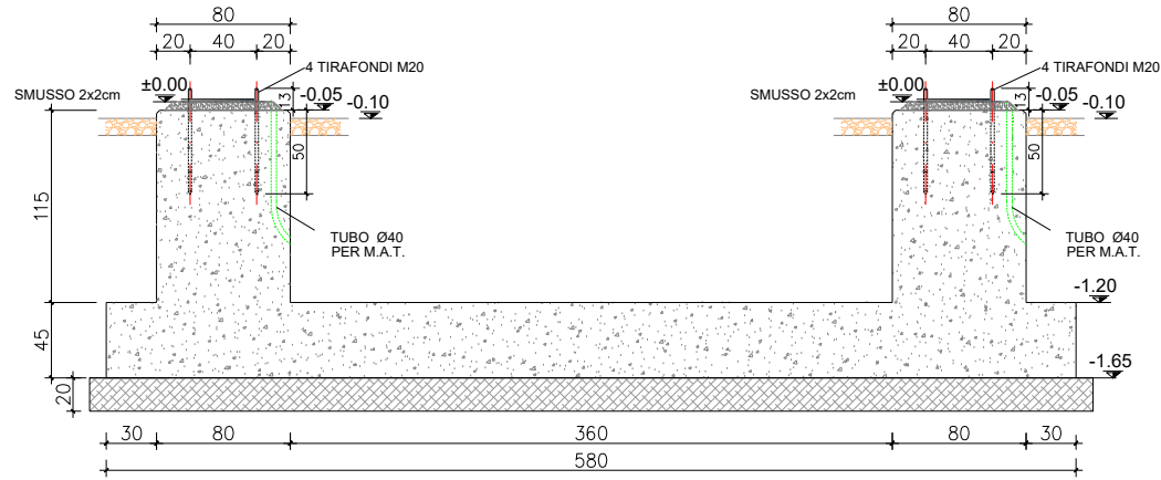
SEZIONE A-A
