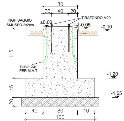
SEZIONE B-B
