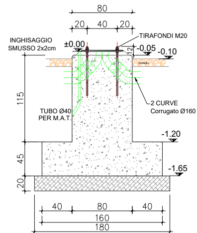
SEZIONE B-B TV
