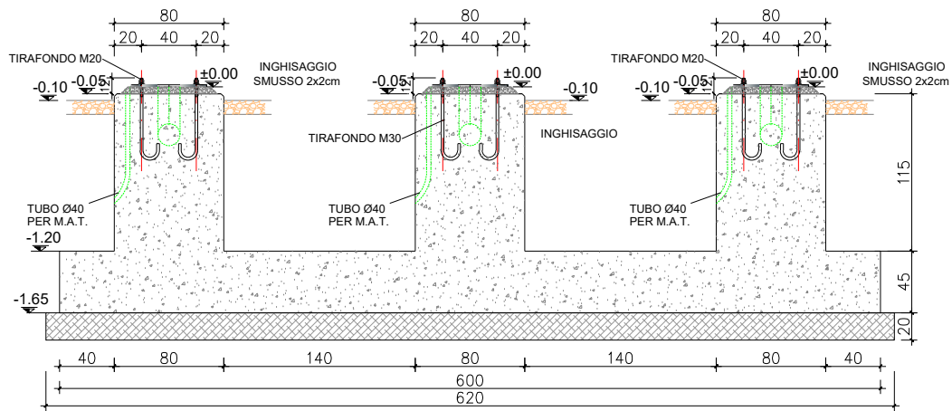
SEZIONE A-A
