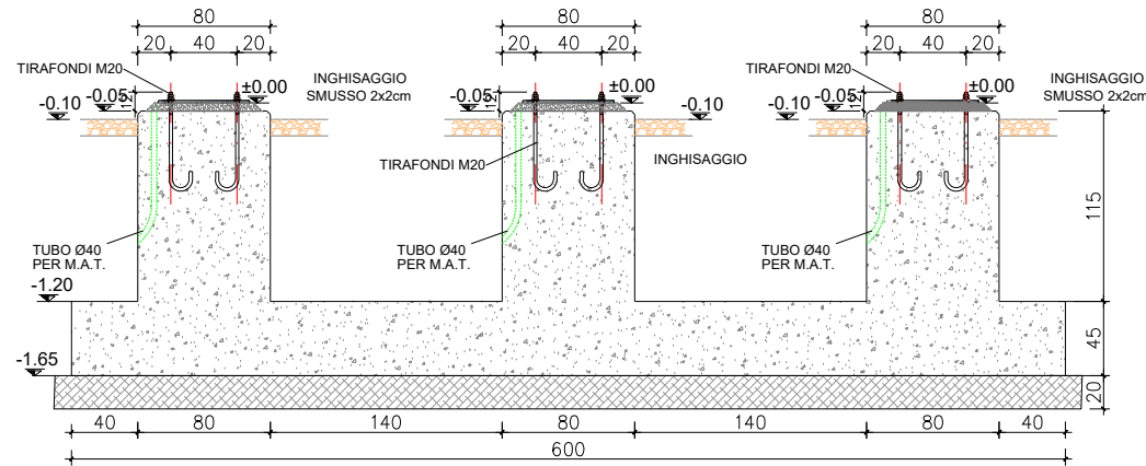
SEZIONE A-A
