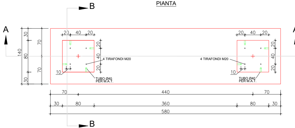
PIANTA
